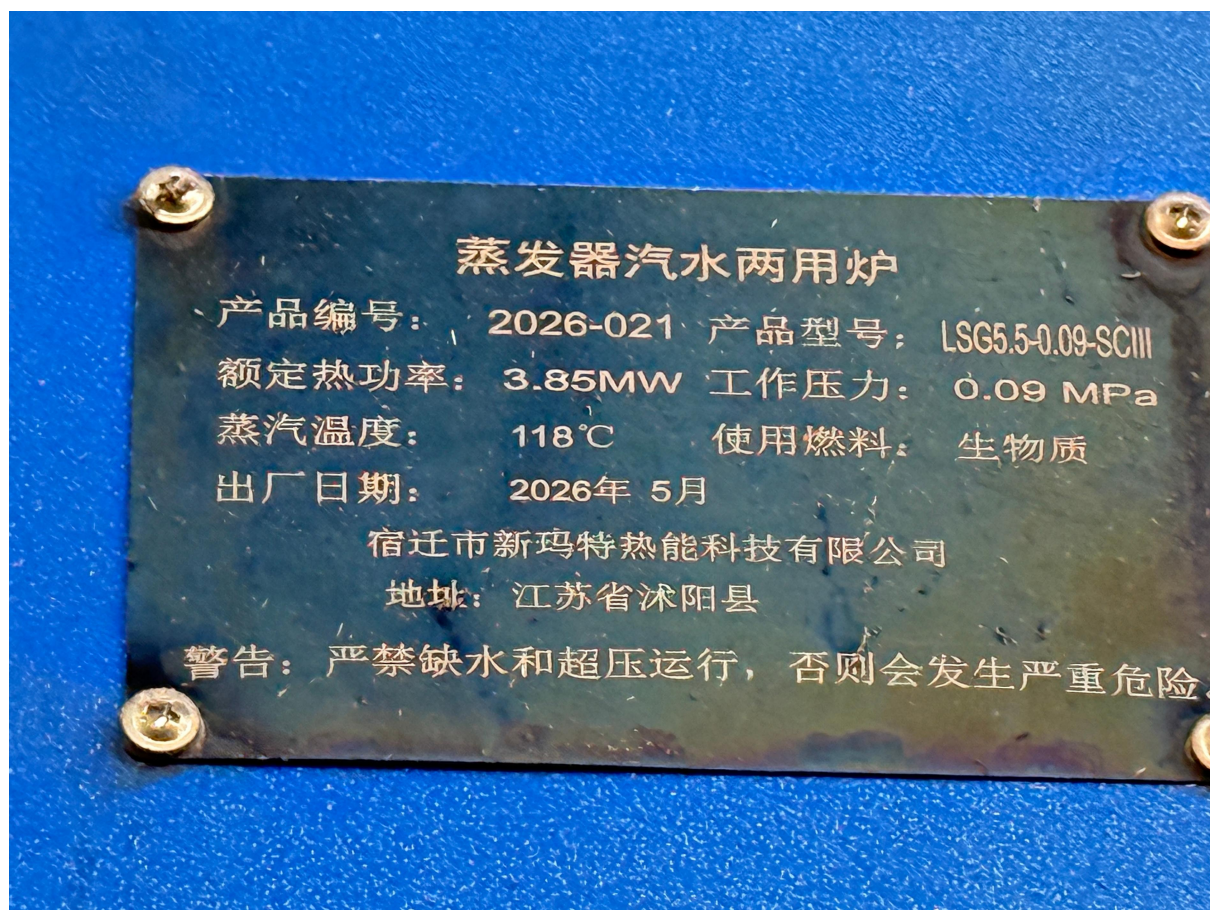
附图 6 项目 5.5t/h 生物质蒸汽发生器铭牌
