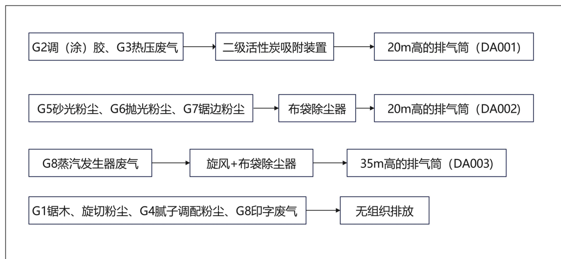
图 2-4 各废气污染源对应污染治理措施流程图
