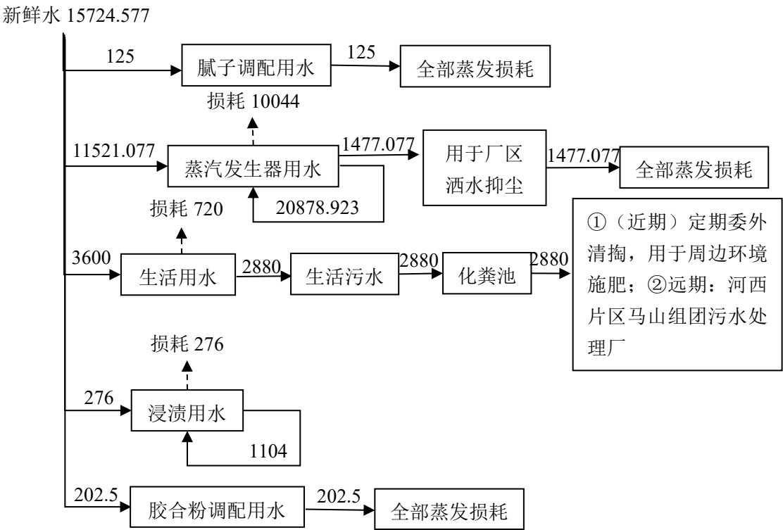
图 2-1 项目水平衡图（单位：m³/a）
