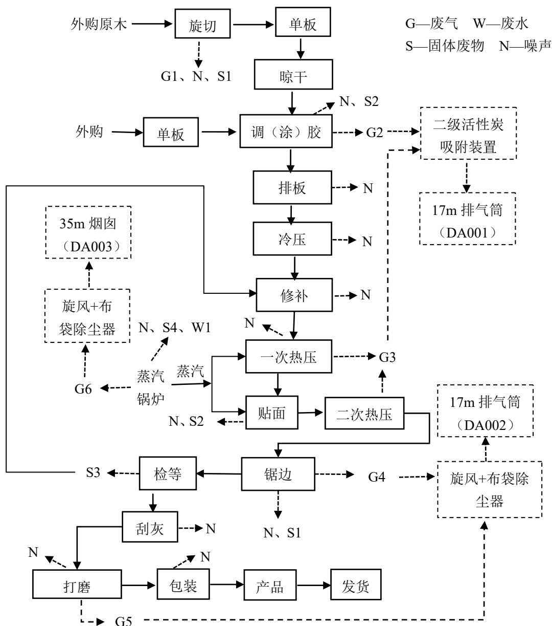
图2-3 项目运营期多层胶合板生产工艺流程及产污环节图
