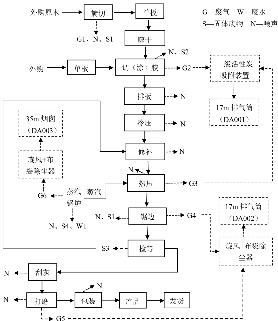
图2-4 项目运营期生态板生产工艺流程及产污环节图
