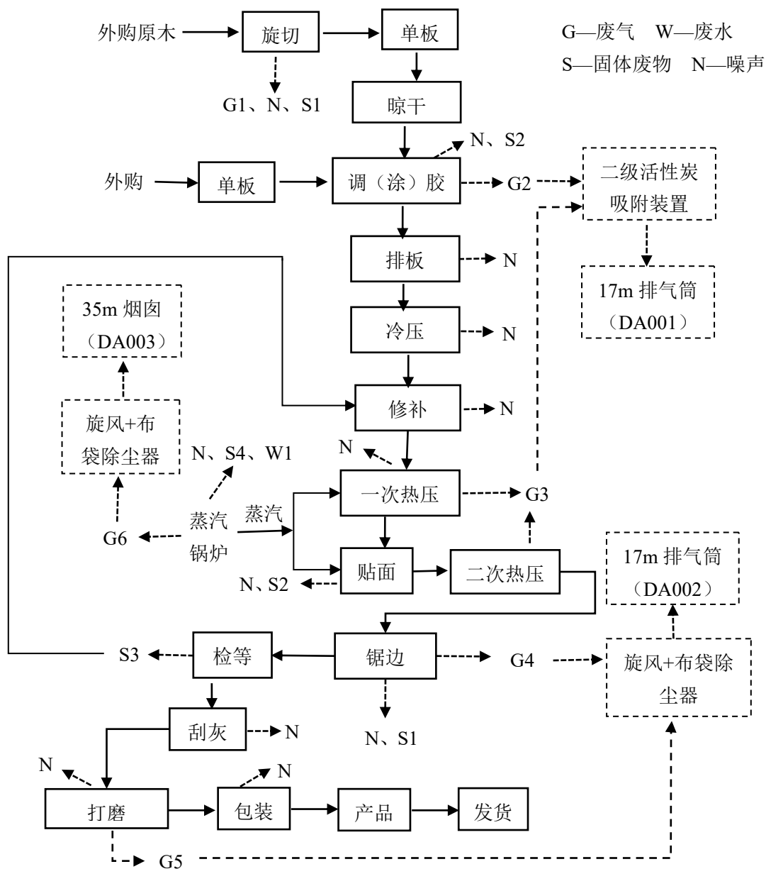
图3.1-2 项目运营期多层胶合板生产工艺流程及产污环节图
