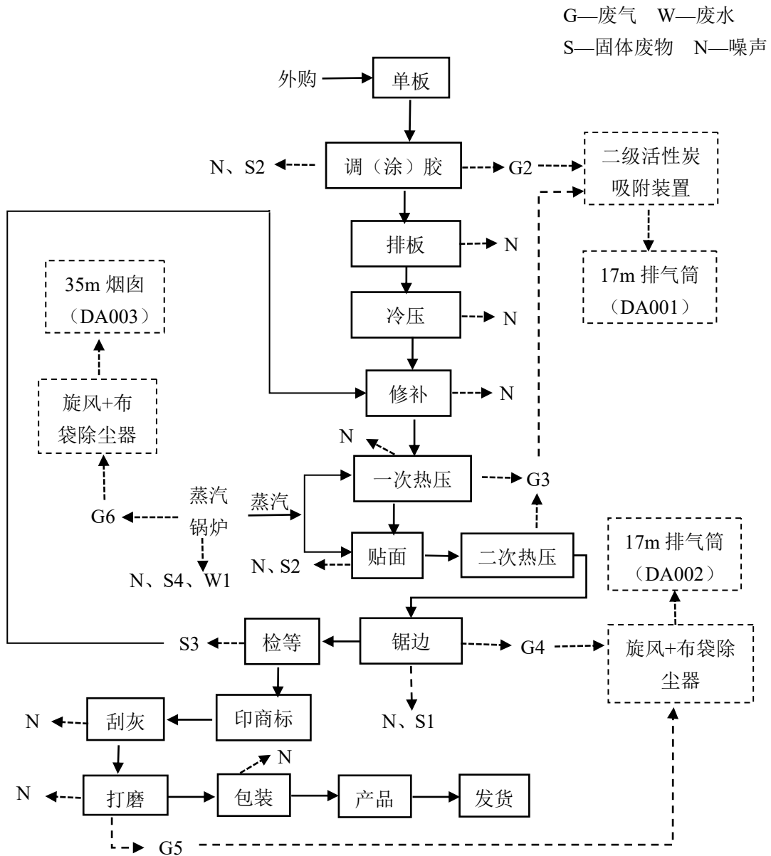
图2-5 项目运营期阻燃板生产工艺流程及产污环节图
