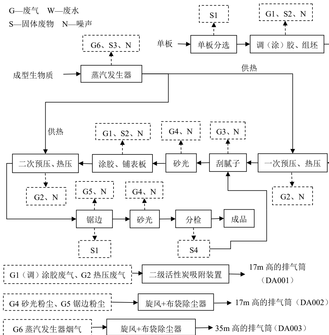
图3.1-2 项目运营期生产工艺流程及产污环节图
