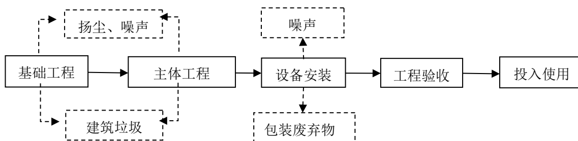
图 3.1-1 项目施工期流程及产污环节图
