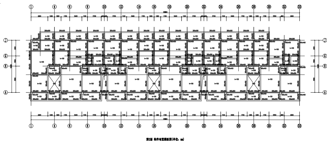
图 5.1.8 三层结构平面图
