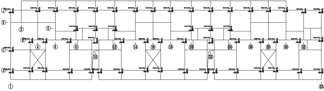
第 5 层（标准层）柱、墙轴压比长度关系简图 \alpha/b ：柱/墙长度/计算单元长度关系 柱按左数时，数值： \alpha/b 上 \alpha/b 下 注：当柱在一个方向截面内时，按左数方向轴压比长度关系，第一个方向轴压比长度
