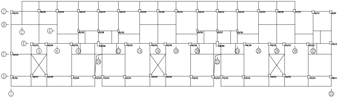
第 3 层 (6683) 抗震验算结果 第 1 层 X向 抗震验算结果=15.3 抗震验算结果=15.3 Y向 抗震验算结果=19.5 抗震验算结果=19.5
