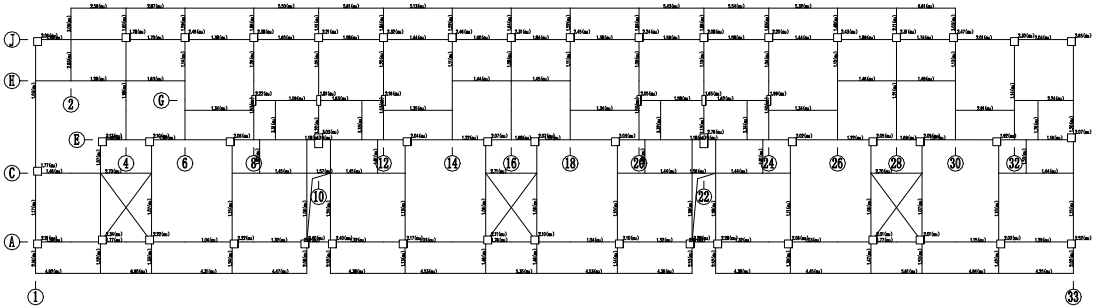
图 5.2.10 一层柱、二层梁安全评级结果简图 (抗力与荷载效应之比)
