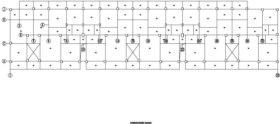
图 5.2.21 四层板安全评级结果简图（抗力与荷载效应之比）
