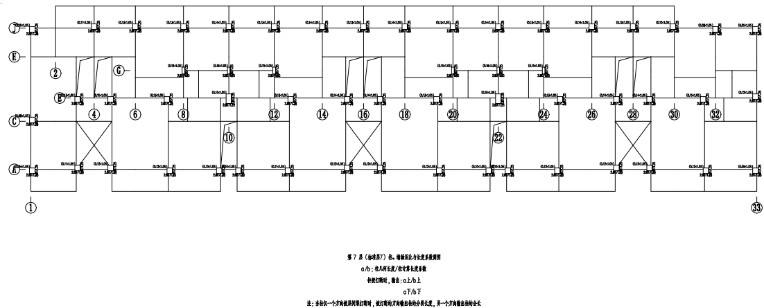
图 5.2.7 七层柱轴压比简图
