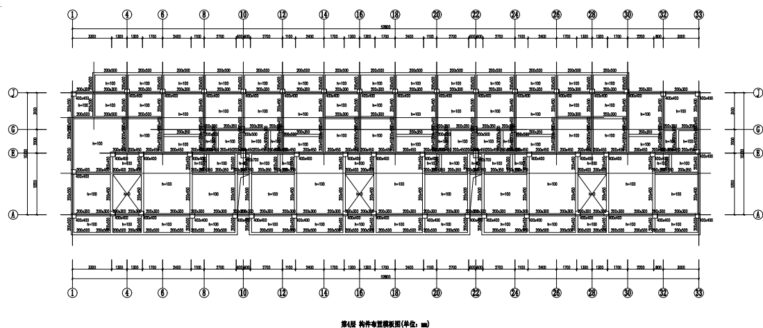
图 5-1-10 五层结构平面图
