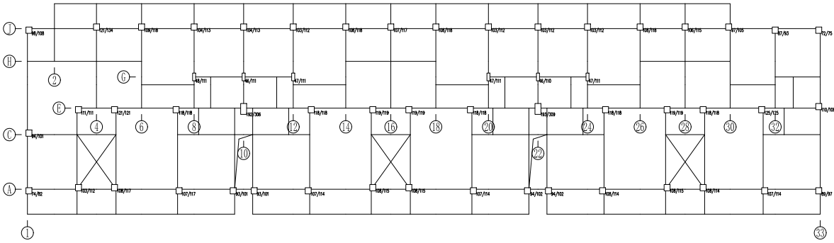
第 5 层 (6685) 抗震验算结果 第 1 层 X向 抗震验算结果=15.8 抗震验算结果=15.8 Y向 抗震验算结果=20.0 抗震验算结果=20.0
