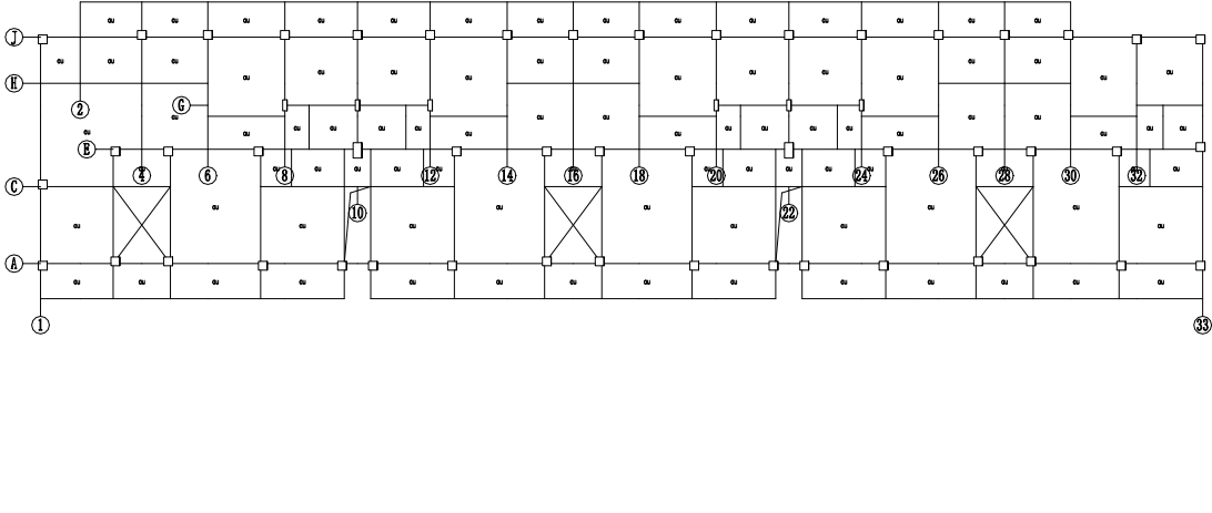
图 5.2.22 五层板安全评级结果简图（抗力与荷载效应之比）
