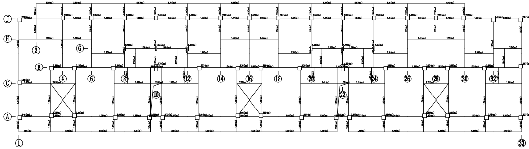
第 4 层 (标准层) 构件安全等级结果图 (承载力控制)
