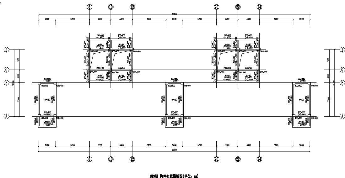
图 5-1-15 屋面构架层结构平面图
