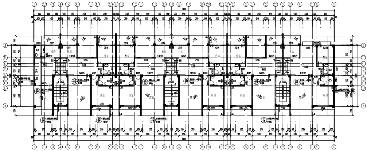
图 5.1.5 八层建筑平面图
