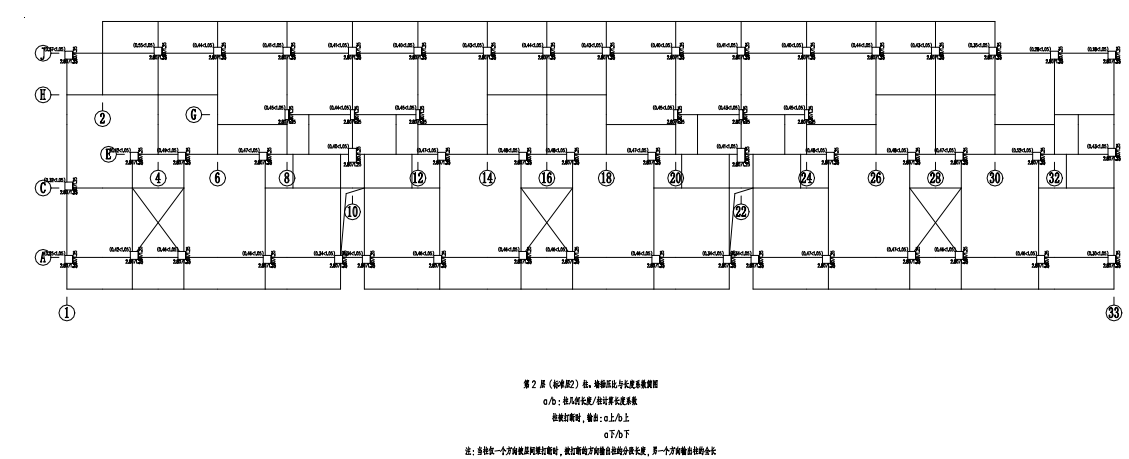
图 5.2-2 二层柱轴压比简图
