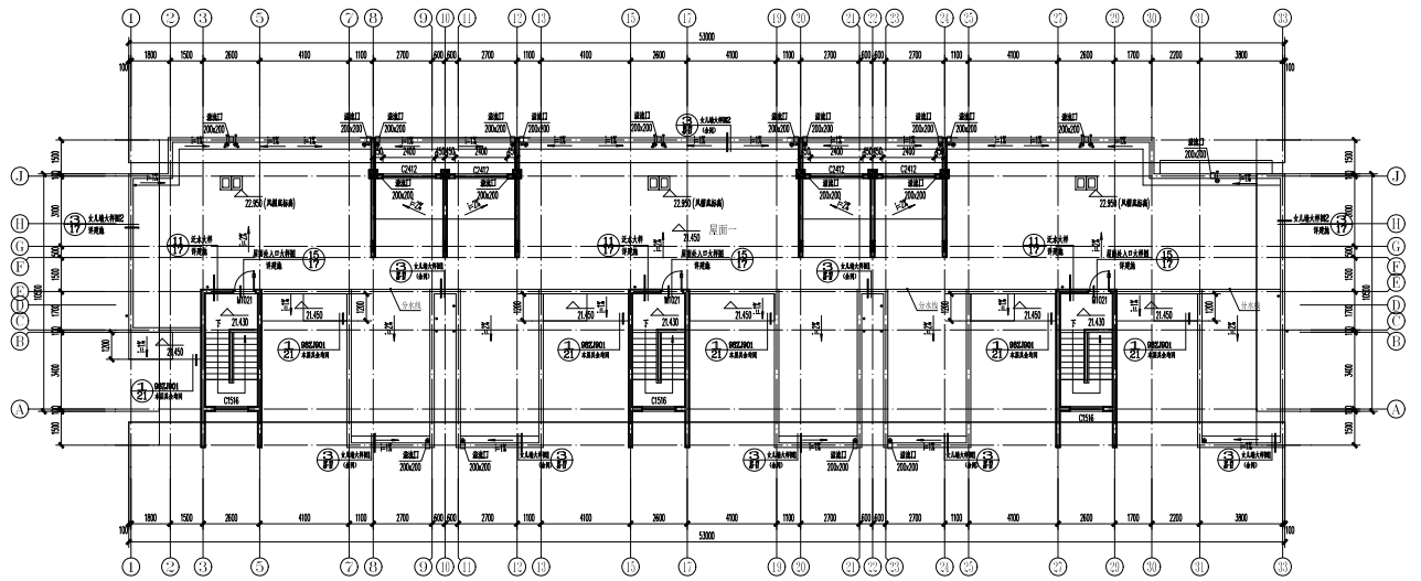
图 5.1.6 屋面层建筑平面图
