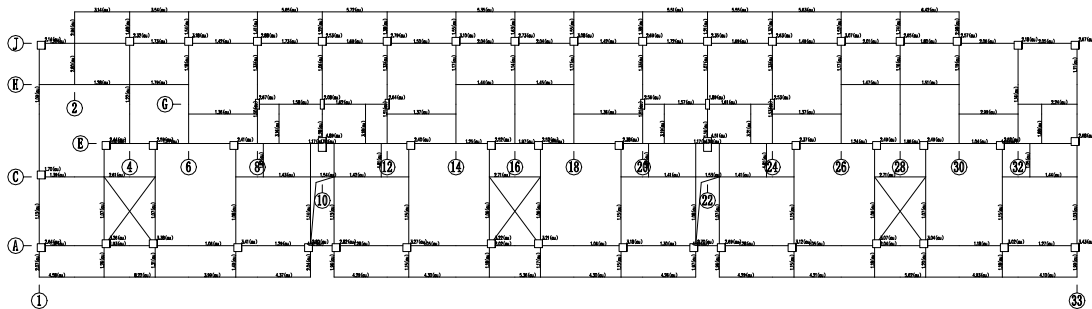
第 5 层 (标准层) 构件安全等级结果图 (承载力控制)
