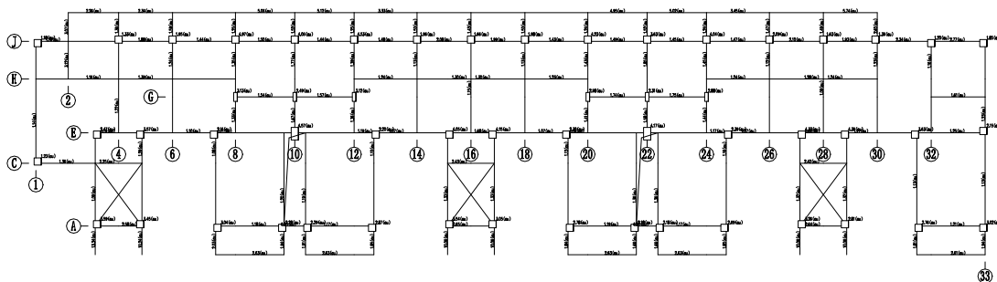
第 8 层 (标准层8) 构件安全评级结果图 (承载力分项)
