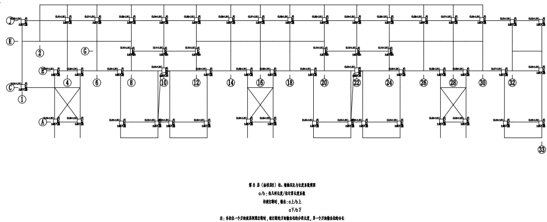
图 5.2.8 八层柱轴压比简图
