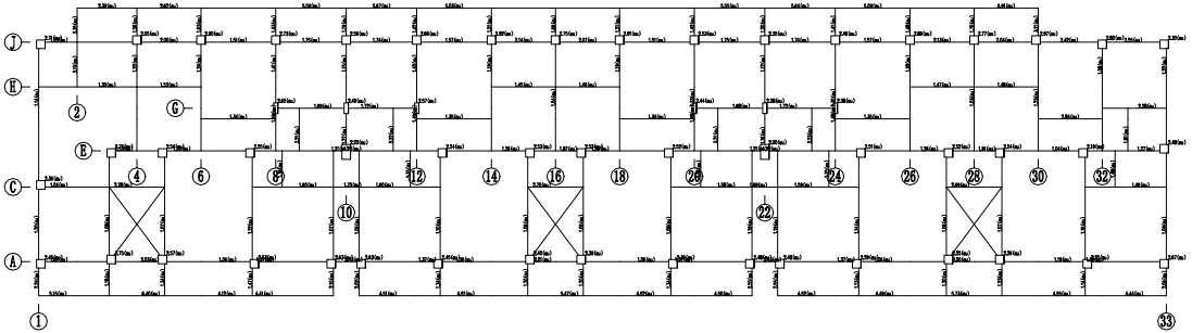
第 1 层 (标准层1) 构件轴压比简图 (未截断柱墙)
