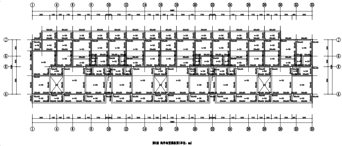
图 5-1-11 六层结构平面图
