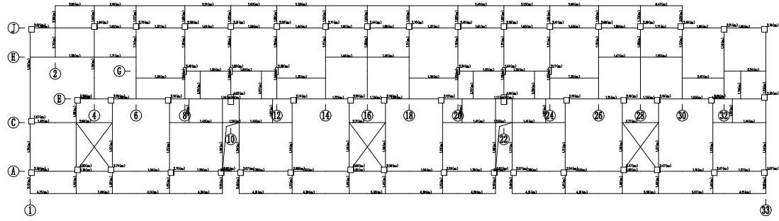
第 3 层 (标准层) 构件安全等级结果图 (承载力控制)
