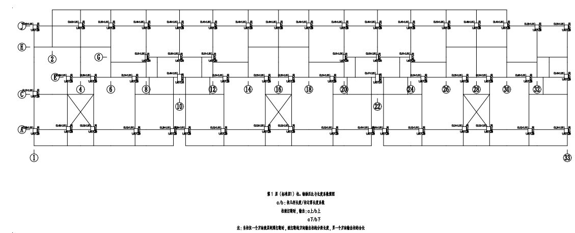
图 5.2.1 一层柱轴压比简图
