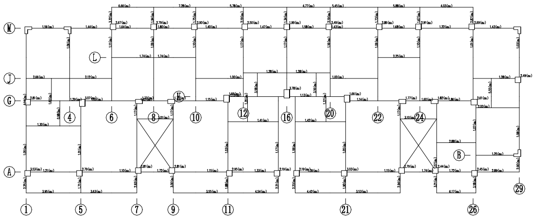
图 5.2.11 二层柱、三层梁安全评级结果简图 (抗力与荷载效应之比)
