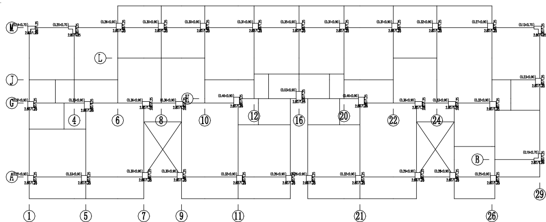
图 5.2.3 三层轴压比简图
