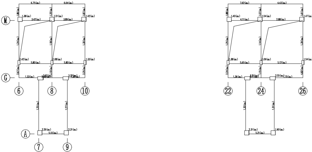
图 5.2.17 八层柱、屋面梁安全评级结果简图 (抗力与荷载效应之比)
