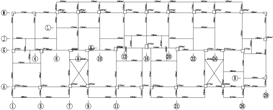
图 5.2.13 四层柱、五层梁安全评级结果简图 (抗力与荷载效应之比)
