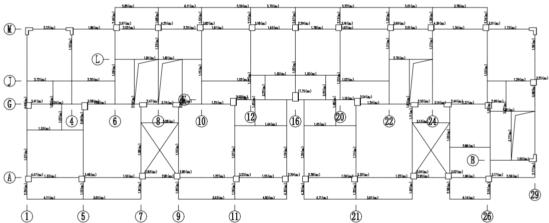
图 5.2.15 六层柱、七层梁安全评级结果简图 (抗力与荷载效应之比)
