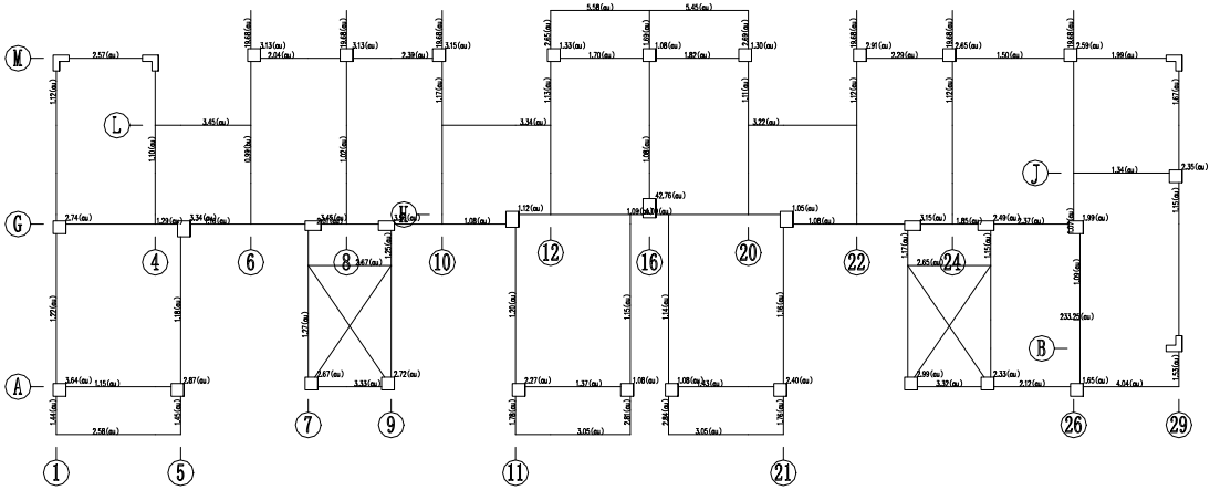
第 8 层 (标准层8) 构件评级结果简图 (承载力项)
