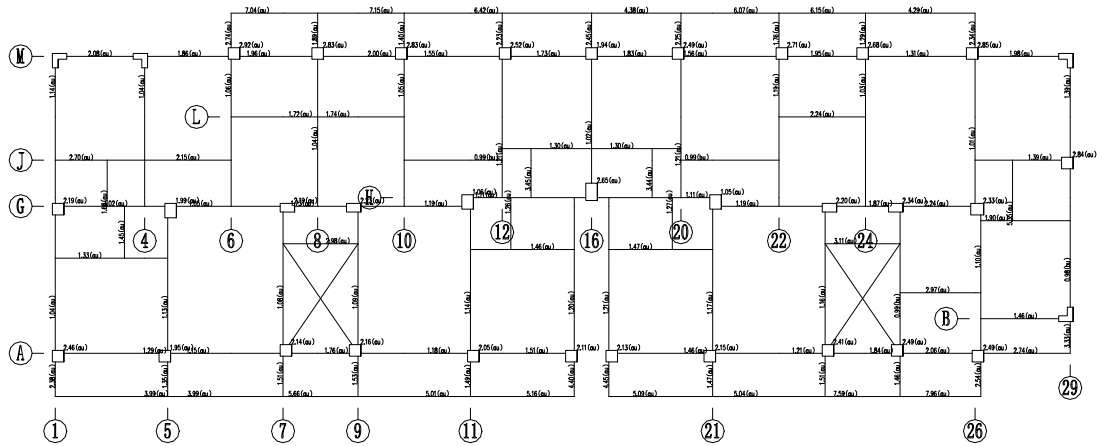
第 1 层 (标准层1) 构件评级结果简图 (承载力分项)
