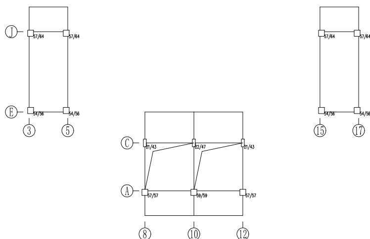
第 9 层 (标准层9) 受弯承载力简图 号: 1 X向 屈服强度系数=33.4 抗震能力指数=33.4 Y向 屈服强度系数=38.1 抗震能力指数=38.1
