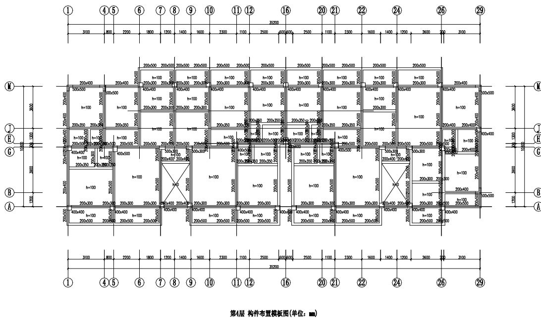
图 5.1.12 五层结构平面图
