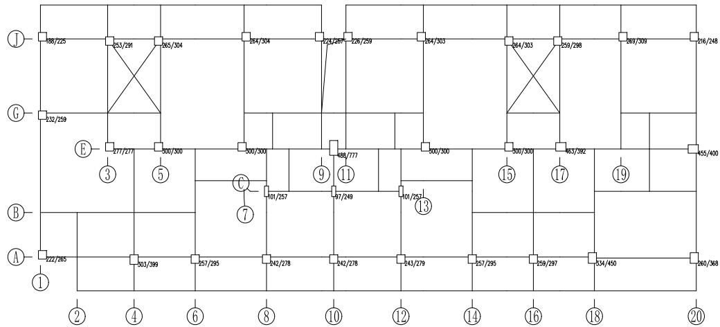
第 1 层 (标准层1) 抗震承载力简图 层数: 1 X 向 屈服强度系数=29.2 抗震能力指数=29.2 Y 向 屈服强度系数=38.1 抗震能力指数=38.1
