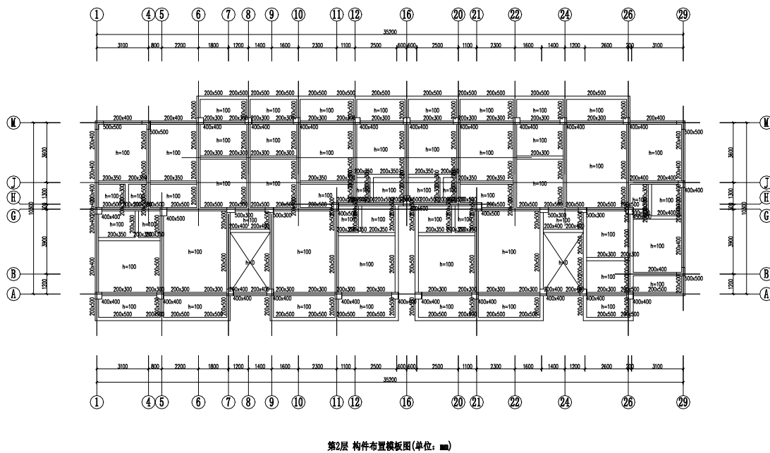
图 5.1.10 三层结构平面图
