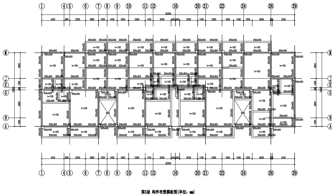
图 5.1.11 四层结构平面图
