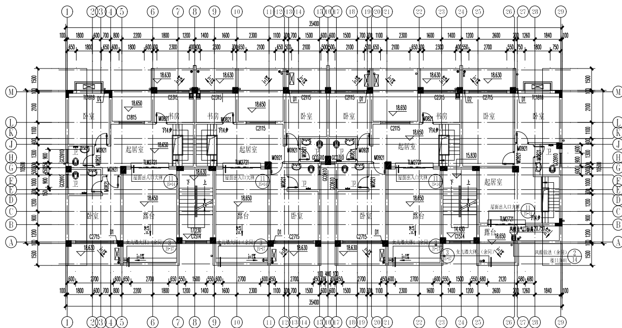
图 5.1.5 七层建筑平面图
