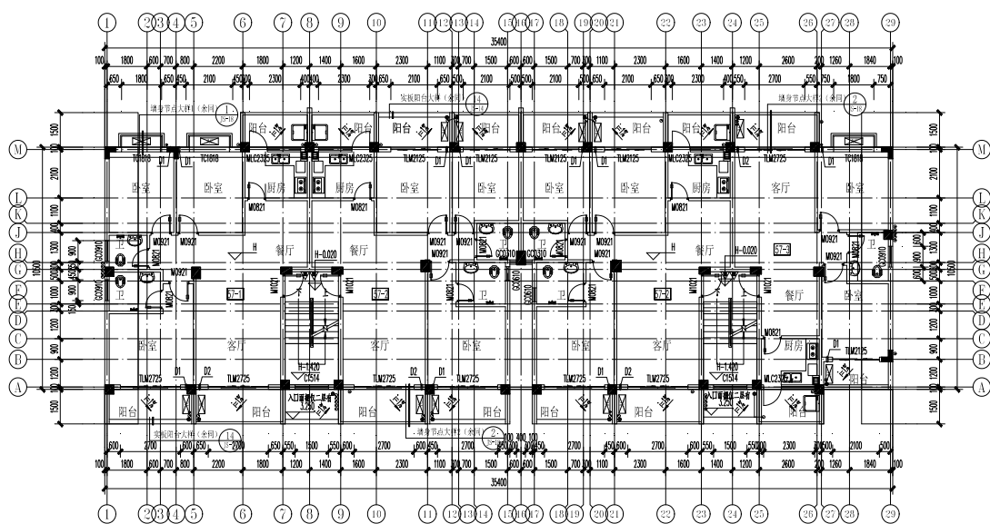
图 5.1.3 二层至五层建筑平面图
