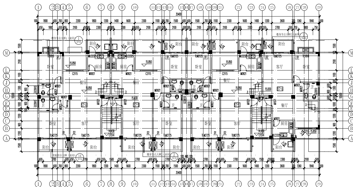
图 5.1.4 六层建筑平面图
