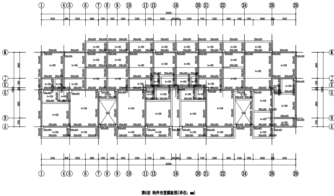
图 5.1.13 六层结构平面图
