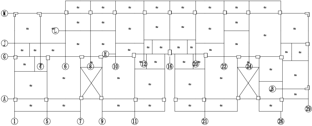
图 5.2.21 四层板安全评级结果简图 (抗力与荷载效应之比)
