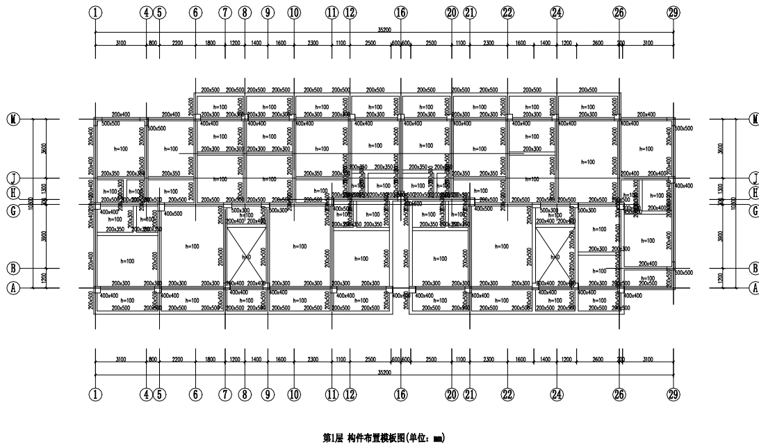
图 5.1.9 二层结构平面图
