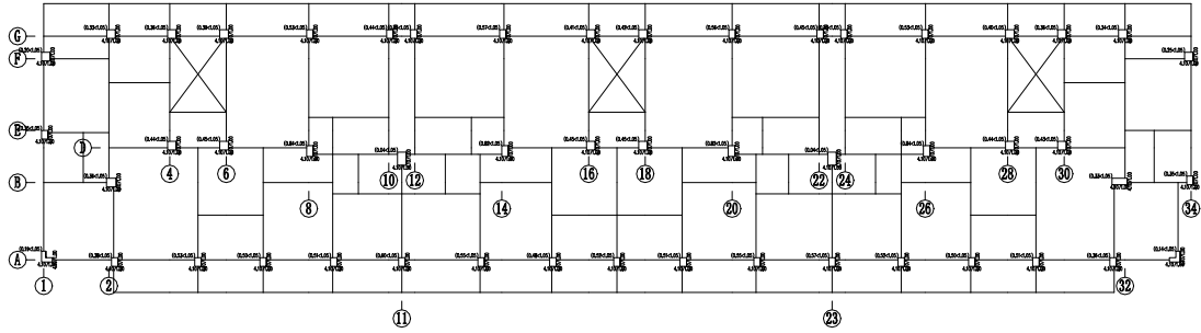
第 1 层 (标准层) 柱、墙轴压比与长度系数简图
