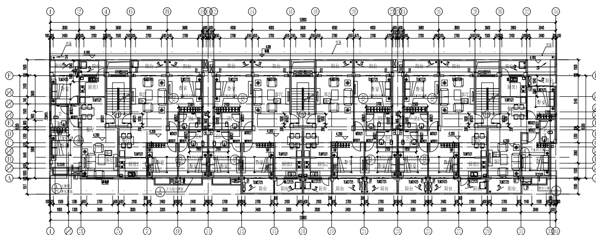
图 5.1.3 二层建筑平面图
