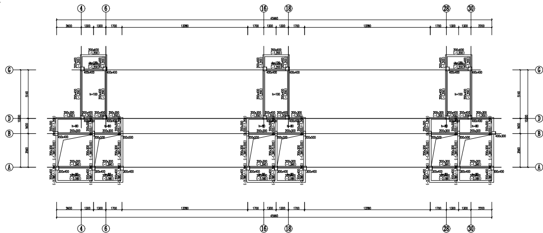
第7层 构件布置模板图(单位: mm)
