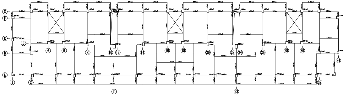
第 6 层 (标准层6) 构件评级结果简图 (承载力分项)
