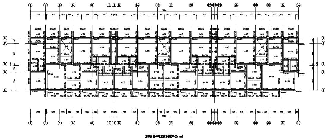
图 5.1.6 二层结构平面图
