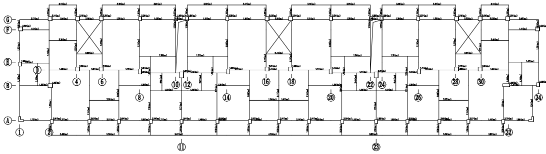
第 3 层 (标准层3) 构件安全评级结果图 (承载力分项)
