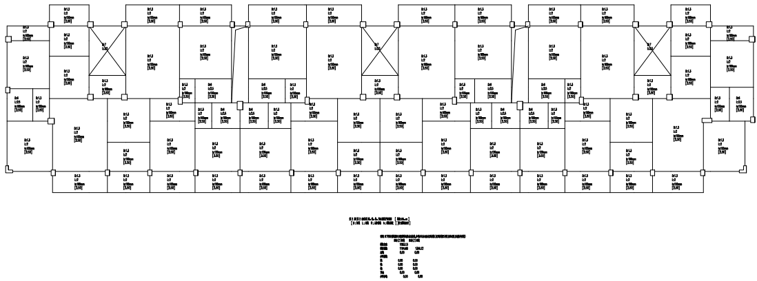
图 5.3.2 二层荷载平面简图
