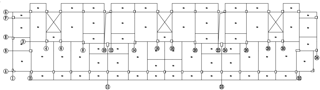
图 5.2.19 六层板安全评级结果简图（抗力与荷载效应之比）
