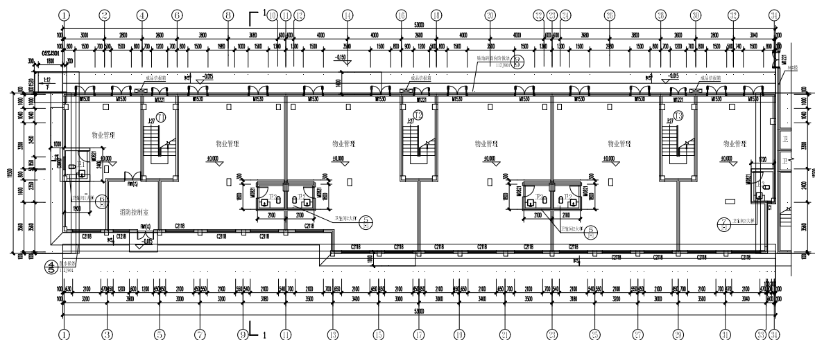
图 5.1.2 一层建筑平面图
