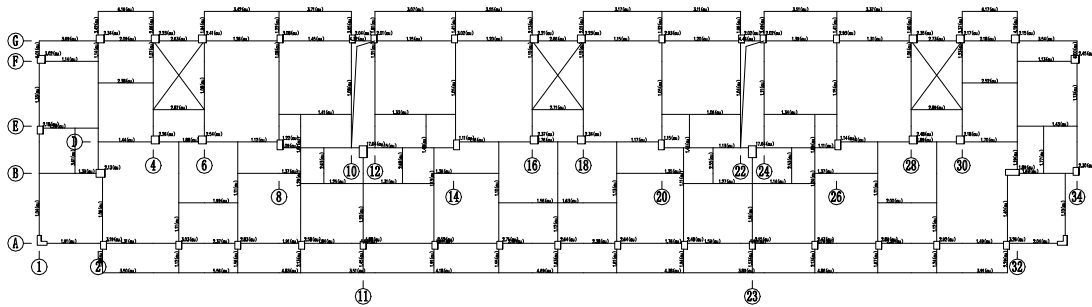
图 5.2.11 四层柱、五层梁安全评级结果简图 (抗力与荷载效应之比)
