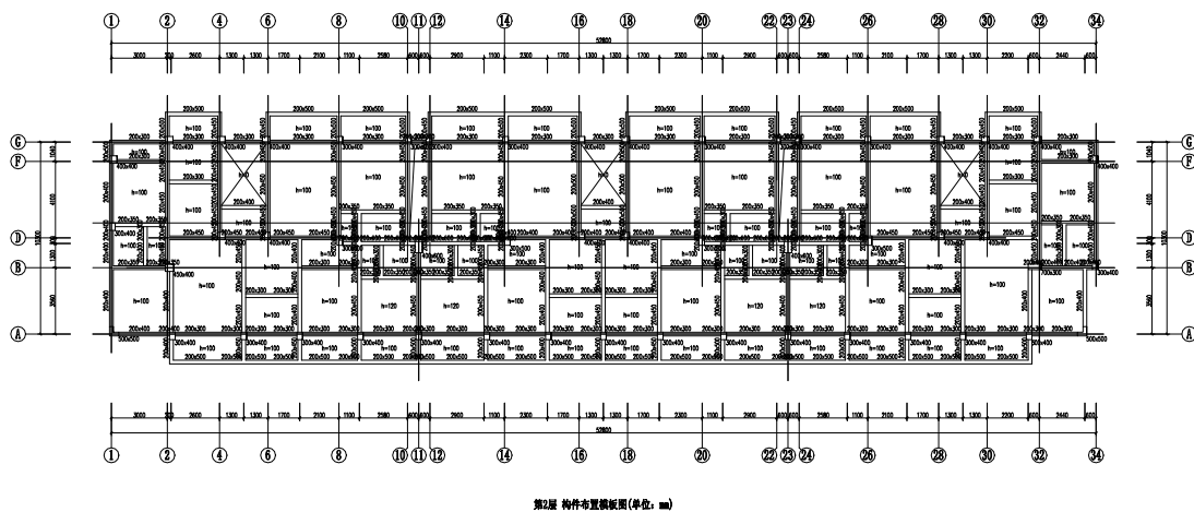
图 5.1.7 三层结构平面图
