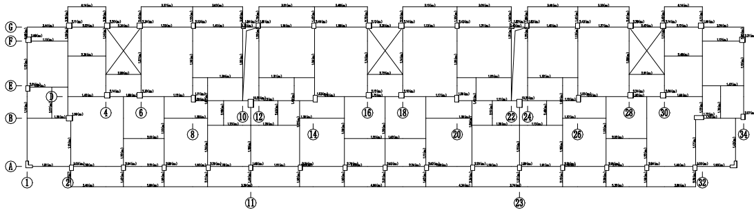
图 5.2.10 三层柱、四层梁安全评级结果简图 (抗力与荷载效应之比)
