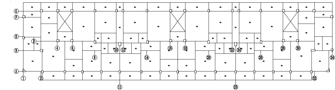
图 5.2.14 七层柱、屋顶构架层梁安全评级结果简图 (抗力与荷载效应之比)
