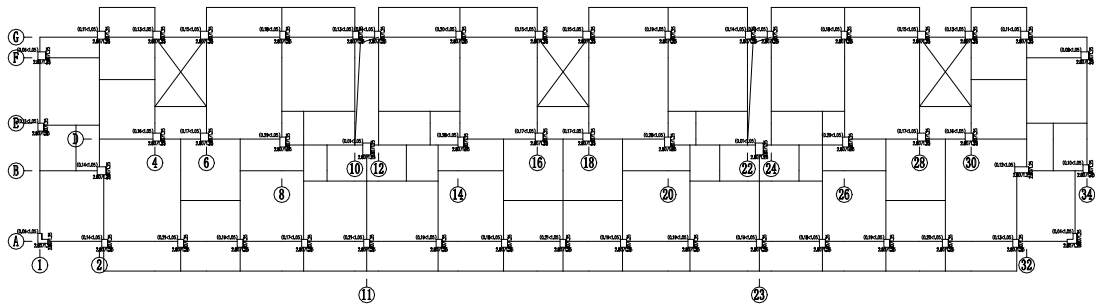
图 5.2.4 四层轴压比简图
