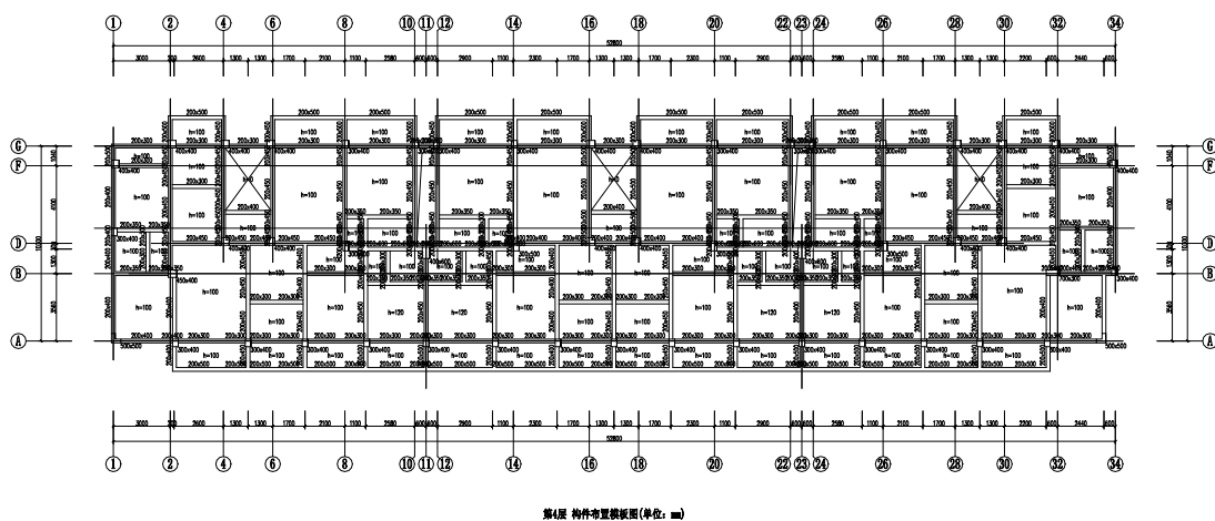
图 5.1.9 五层结构平面图
