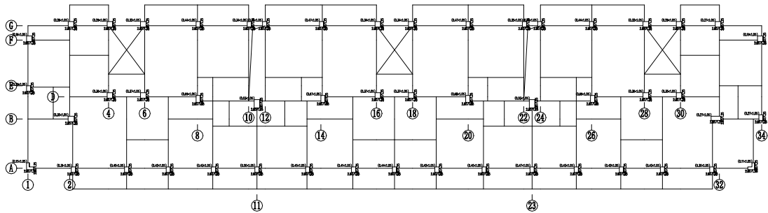
图 5.2.1 一层轴压比简图
