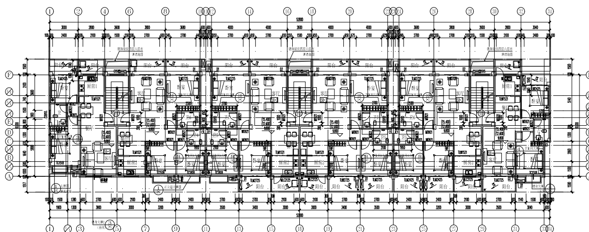
图 5.1.4 三层至六层建筑平面图
