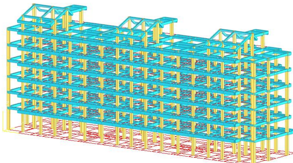
图 5.1.1 建模简图
