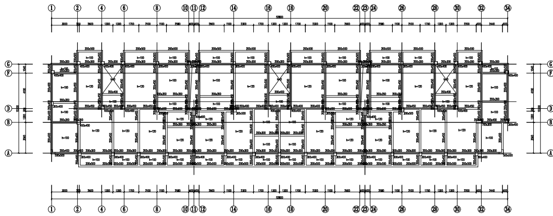
第6层 构件布置模板图(单位: mm)
