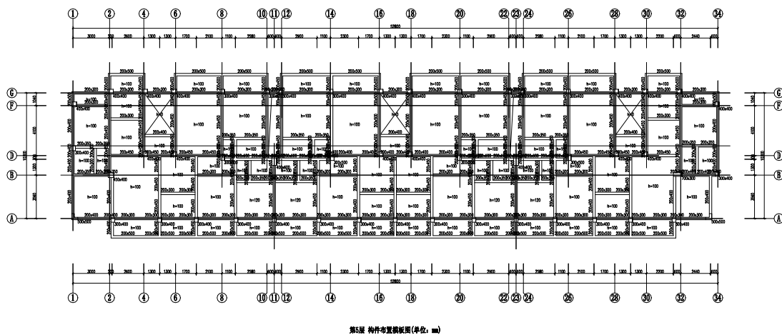
图 5.1.10 六层结构平面图
