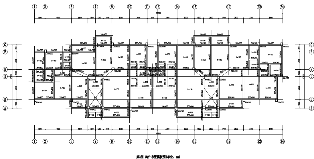
图 5.1.10 B 区三层结构平面图
