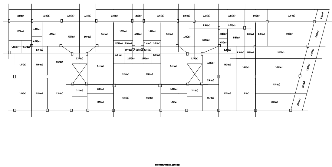
图 5.2.30 B 区二层板安全评级结果简图 (抗力与荷载效应之比)
