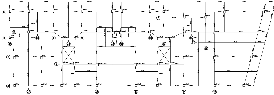
第 1 层 (标准层) 构件评级结果简图 (承载力分项)
