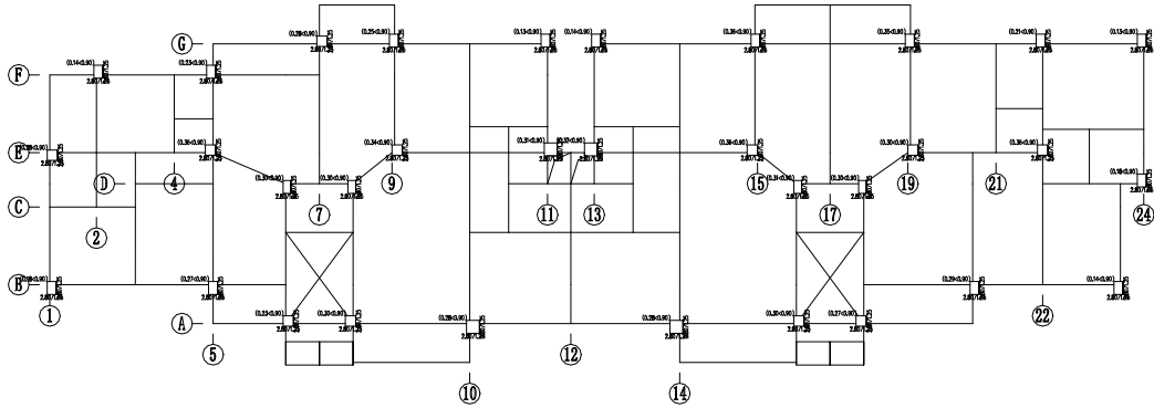
图 3 A (标准层3) 轴压比分布图
