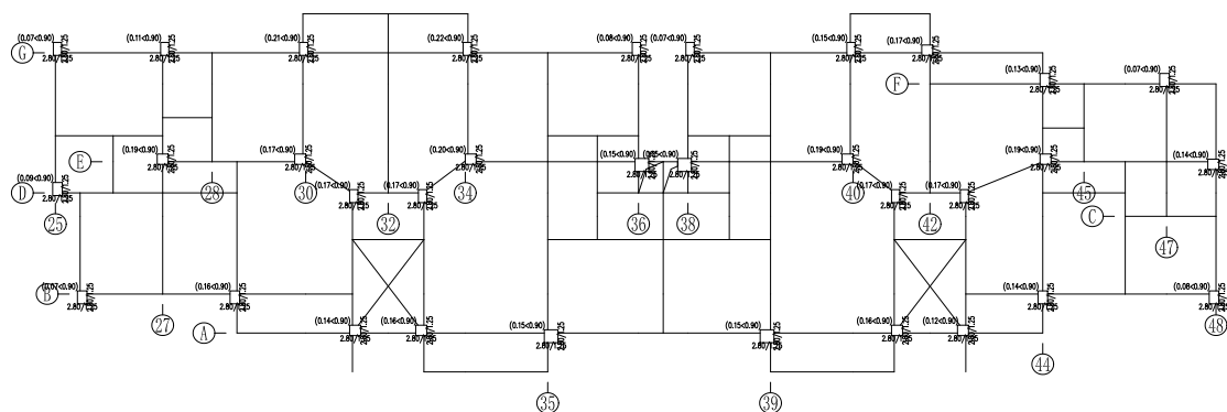
第 5 层 (标准层 5) 墙柱叠柱压比简图
