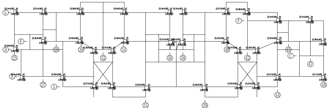
图 5.2.5 A 区三层轴压比简图
