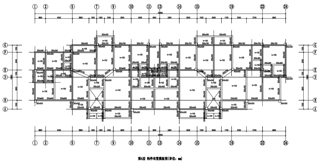
图 5.1.12 B 区四层结构平面图
