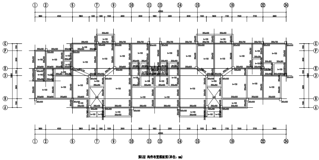
图 5.1.14 B 区五层结构平面图
