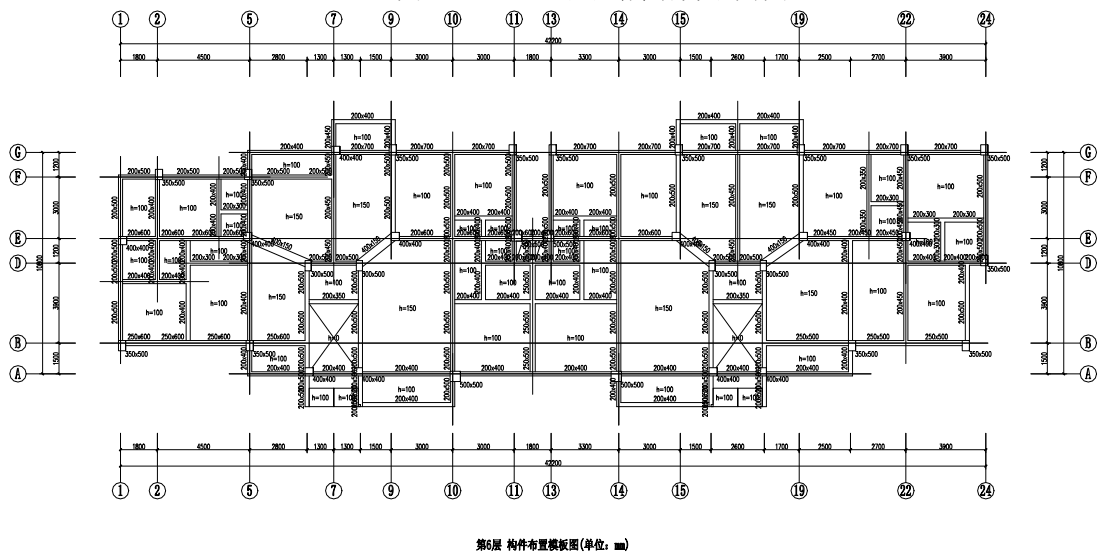
图 5.1.16 B 区六层结构平面图
