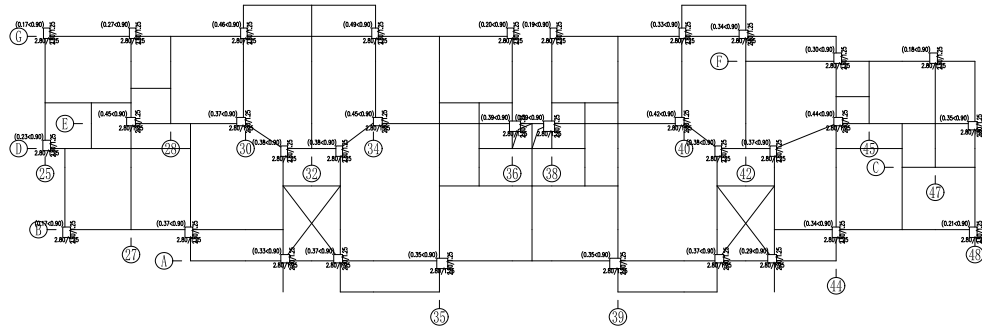
图 2 B (标准层) 轴压比分布图
