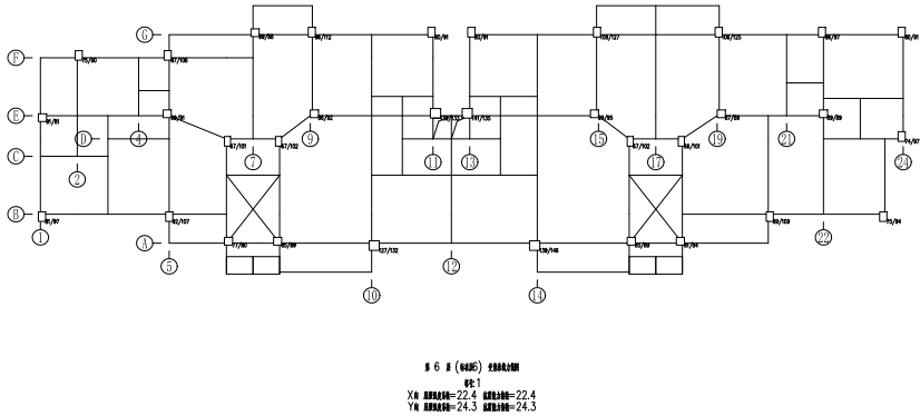
图 6.3.11 A 区六层抗震验算结果
