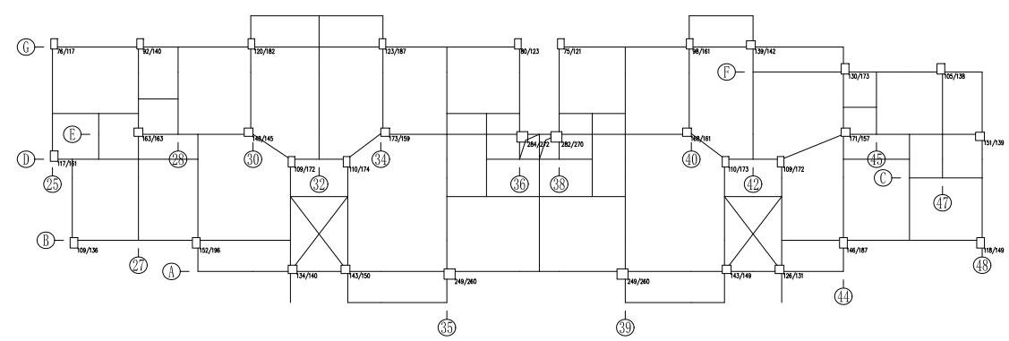
第 2 层 (标准层)(第 2 标准层) 抗震承载力验算 单元: 1 X 向 抗震承载力=13.2 抗震承载力=13.2 Y 向 抗震承载力=16.3 抗震承载力=16.3
