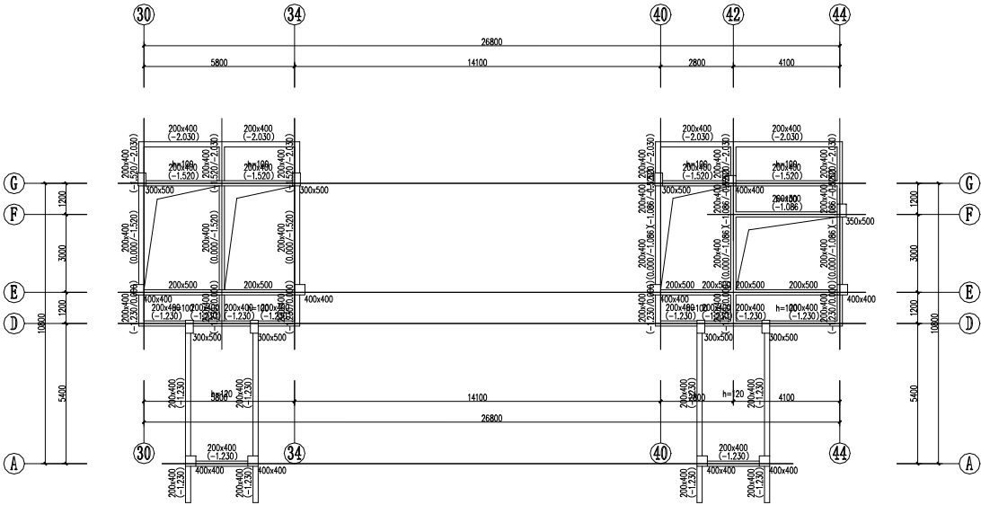
第7层 构件布置模板图(单位: mm)
