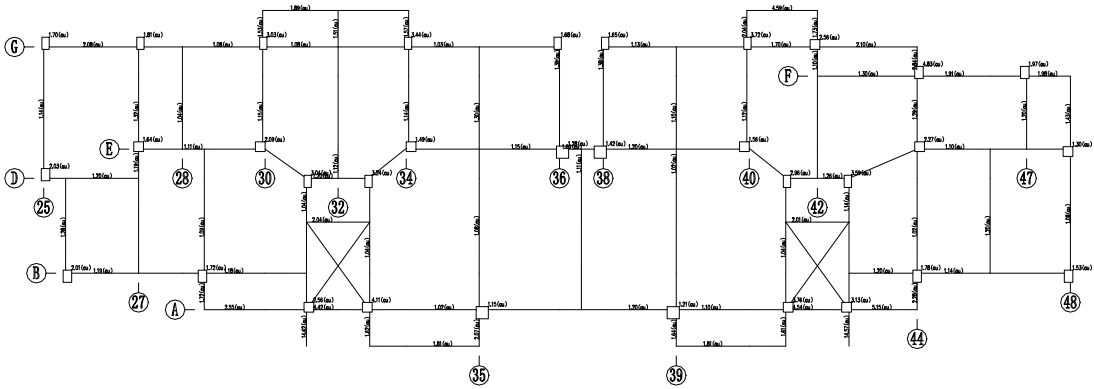
第 6 层 (标准层6) 构件评级结果简图 (承载力项)
