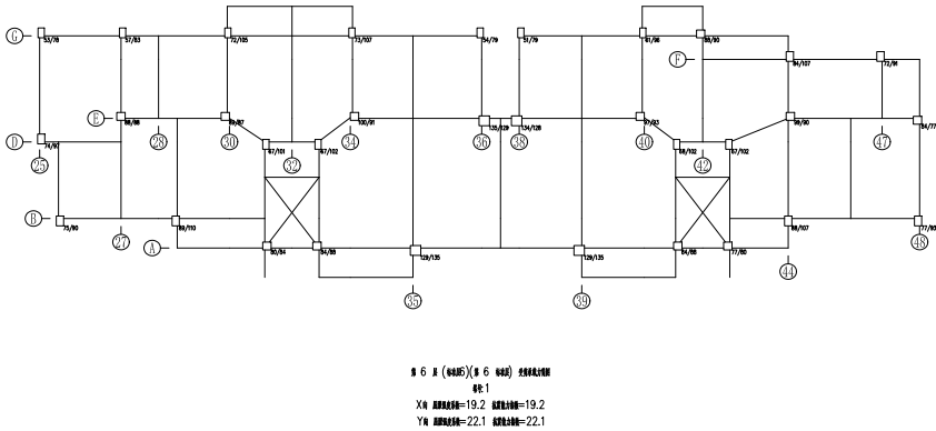
图 6.3.12 B 区六层抗震验算结果
