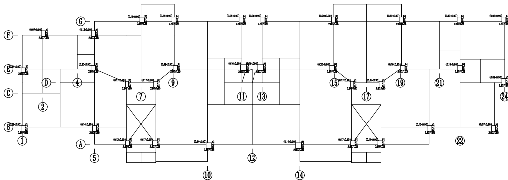
图 5.2.8 B 区四层轴压比简图
