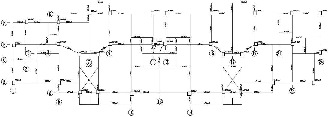
第 4 层 (标准层4) 构件评级结果简图 (承载力分项)
