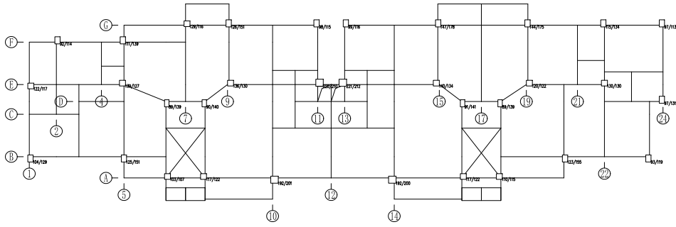
第 4 层 (标准层) 抗震承载力验算 层数: 1 X向 抗震承载力=15.6 抗震承载力=15.6 Y向 抗震承载力=18.9 抗震承载力=18.9
