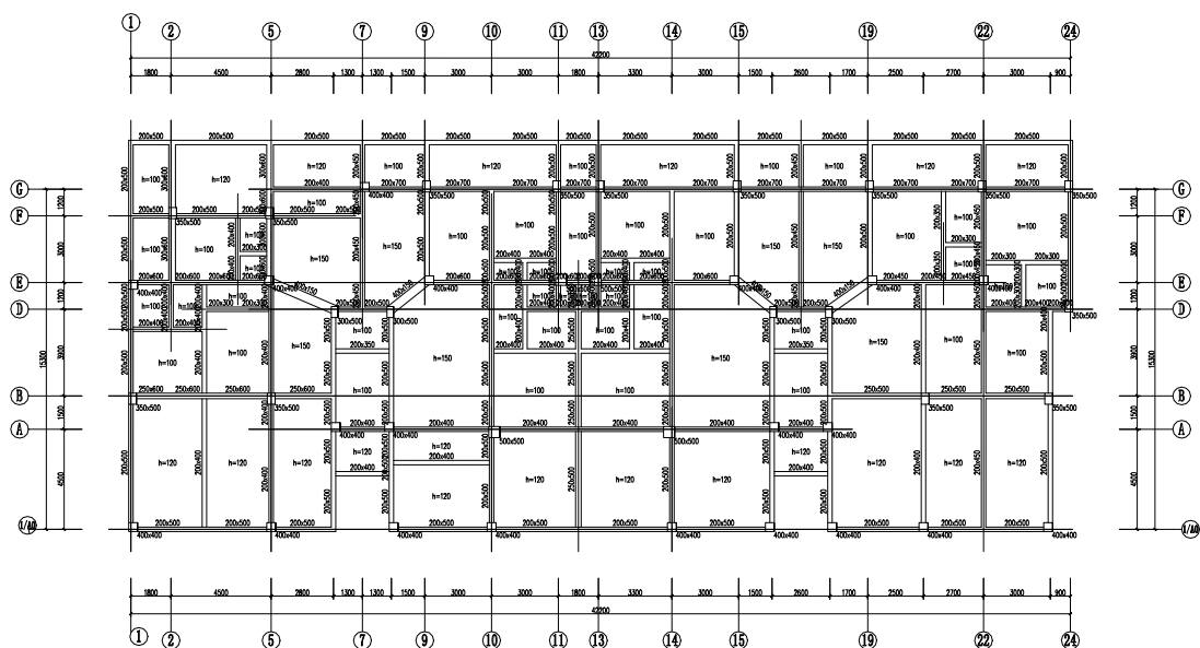
第1层 构件布置模版图(单位: mm)
