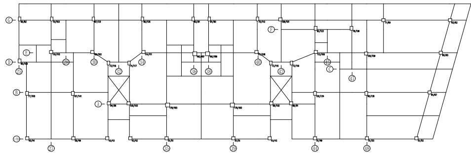
图 6.3.1 A 区一层抗震验算结果
