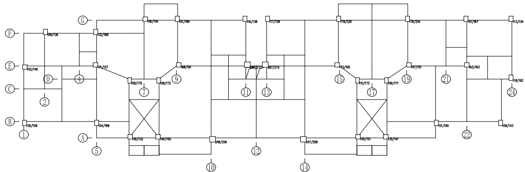
图 6.3.2 B 区一层抗震验算结果
