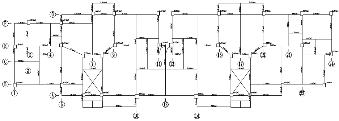
第 3 层 (标准层3) 构件评级结果简图 (承载力分项)
