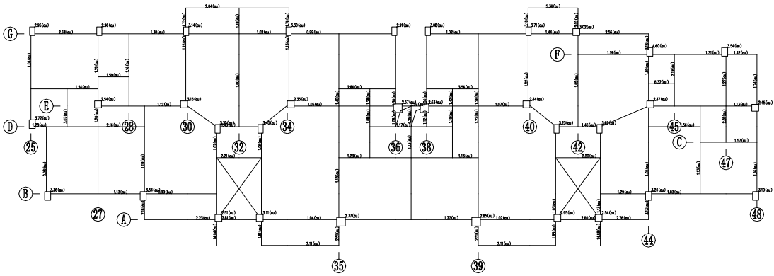
图 5.2.21 A 区四层柱、五层梁安全评级结果简图 (抗力与荷载效应之比)
