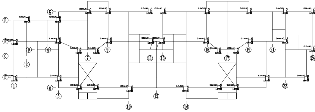
第 4 层 (标准层4) 柱、墙轴压比与长度系数简图 a/b : 柱几何长度/柱计算长度系数 柱被打破时, 输出: a \geq b 上 a < b 下 注: 当柱在一个方向被层间刚度打破时, 被打破的方向输出柱的分配长度, 另一个方向输出柱的全长
