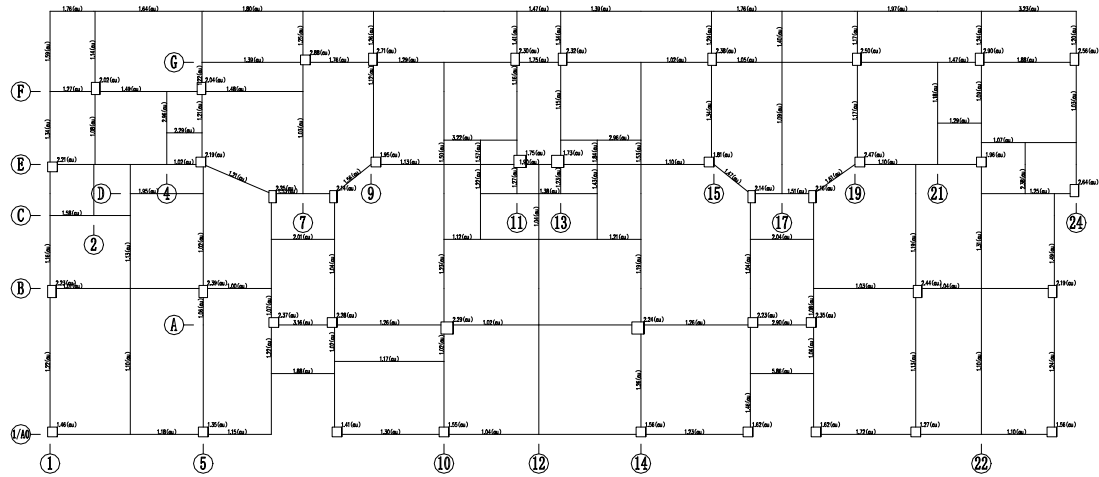
第 1 层 (标准层) 构件评级结果简图 (承载力分项)
