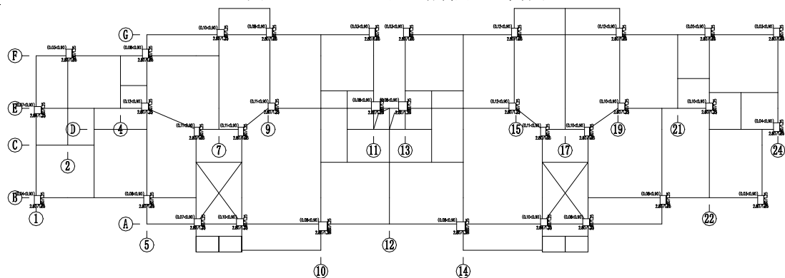
图 5.2.10 B 区五层轴压比简图
