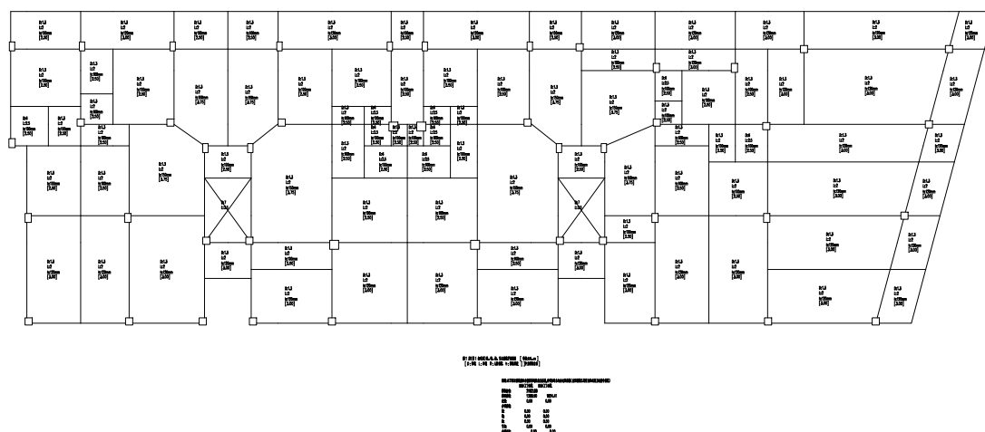
图 5.3.2 B 区一层荷载平面简图
