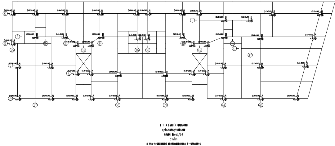
图 5.2.2 B 区一层轴压比简图
