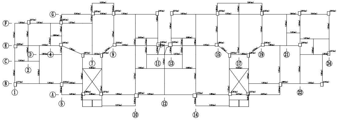
第 2 层 (标准层2) 构件评级结果简图 (承载力项)
