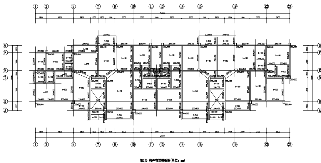
图 5.1.8 B 区二层结构平面图
