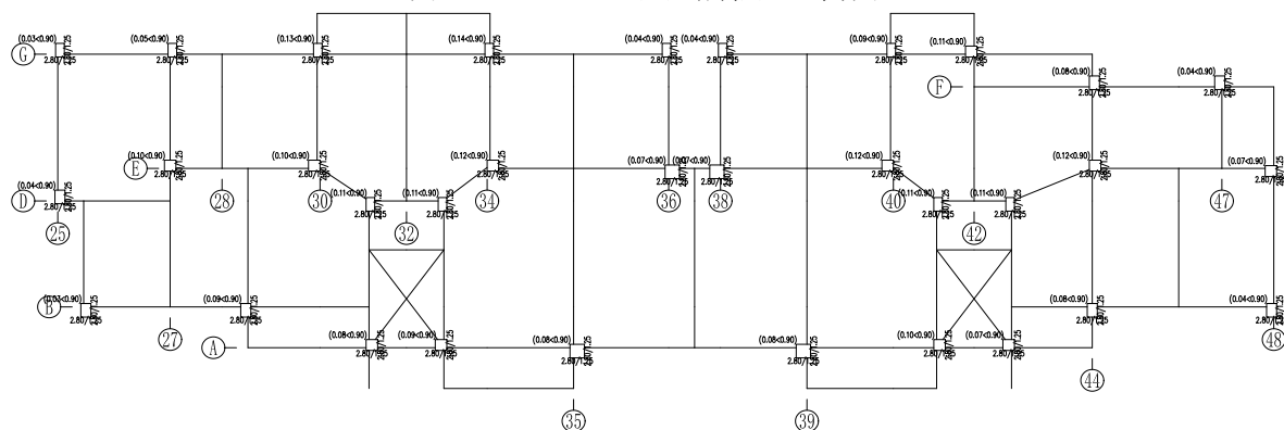
图 5.2.11 A 区六层轴压比简图
