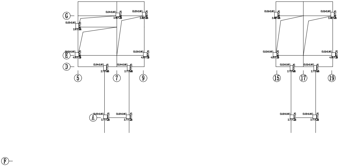
第 7 层（标准层7）柱、墙轴压比与长度系数简图
