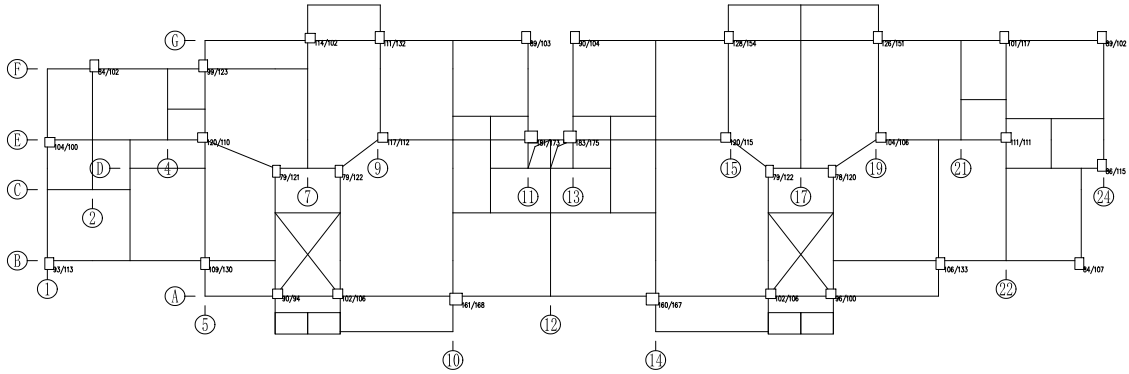
图 6.3.8 B 区四层抗震验算结果
