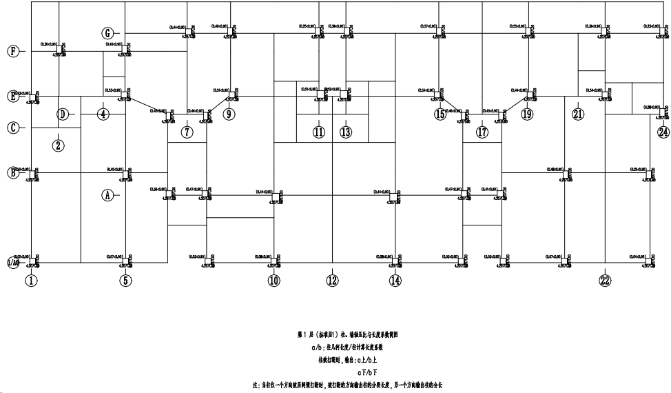
图 5.2.1 A 区一层轴压比简图
