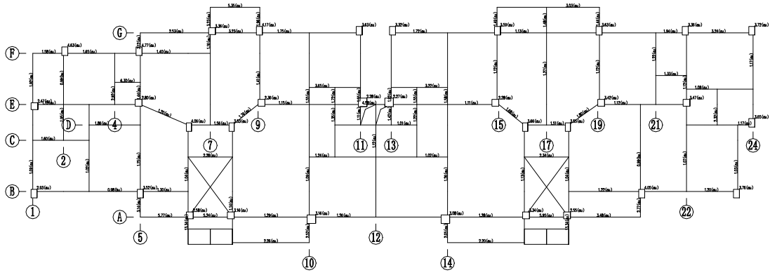
第 5 层 (标准层5) 构件评级结果简图 (承载力分项)
