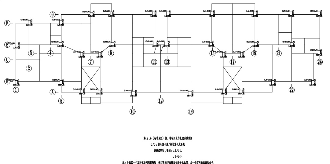
图 5.2.3 A 区二层轴压比简图
