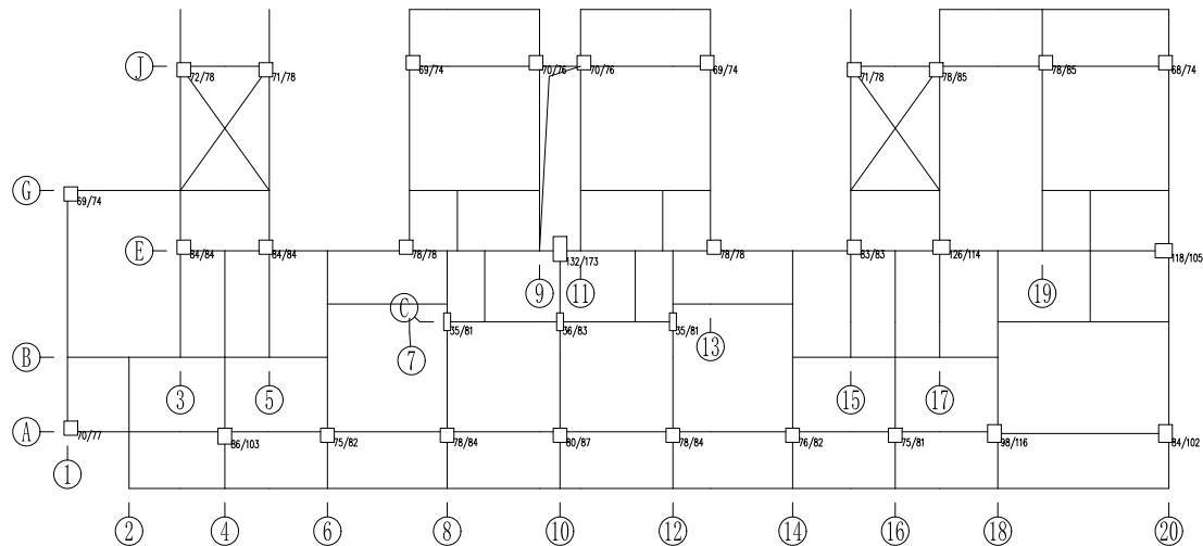
图 6.3.7 七层抗震验算结果
