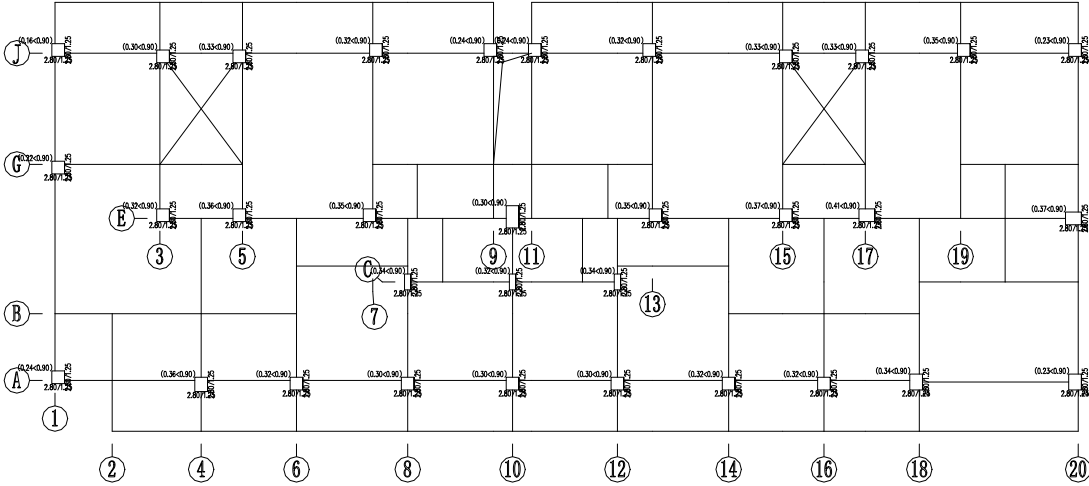
第 4 层（标准层4）柱、墙轴压比与长度系数简图
