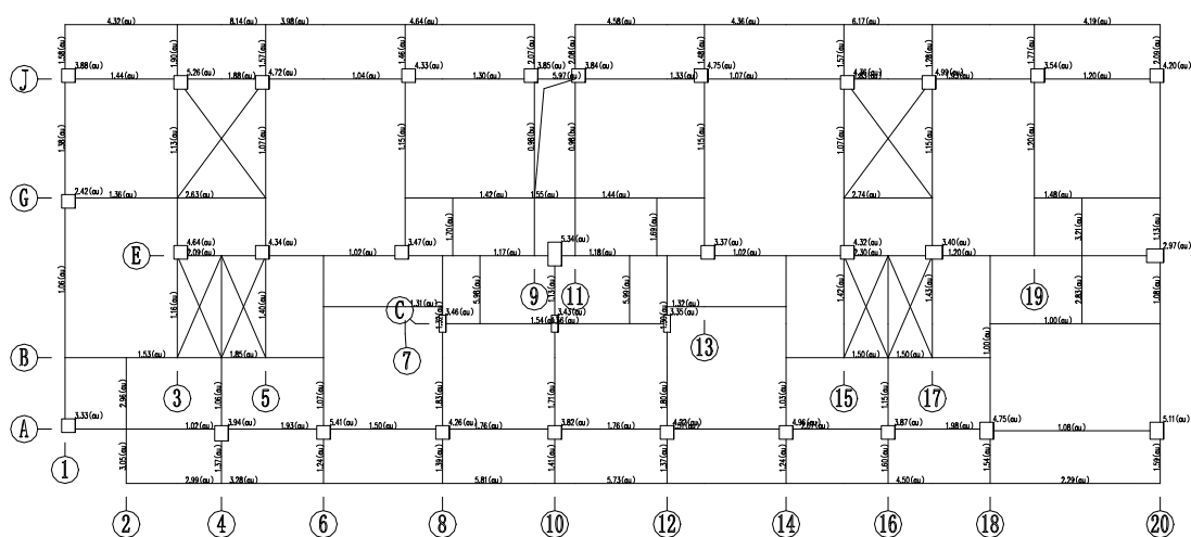
第7层(标准层7)构件评级结果简图(承载能力项)
