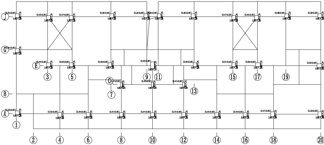
第 2 层 (标准层2) 柱、墙轴压比与长度系数简图
