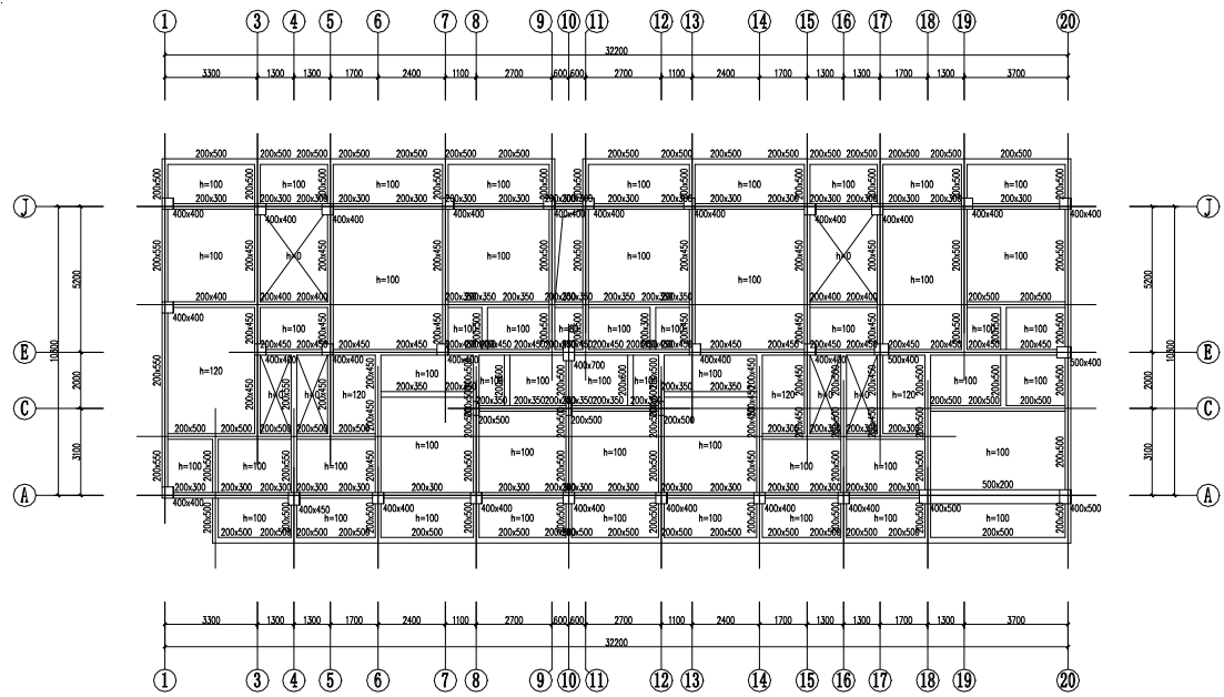
第7层 构件布置模板图(单位: mm)
