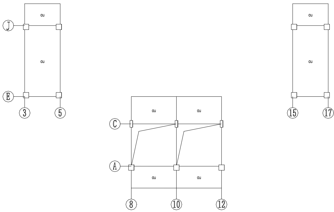
第9层楼面板承载力评级结果图(与面处理包络)
