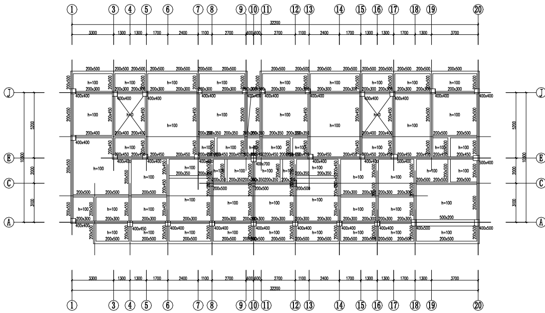
图 5.1.8 二层结构平面图
