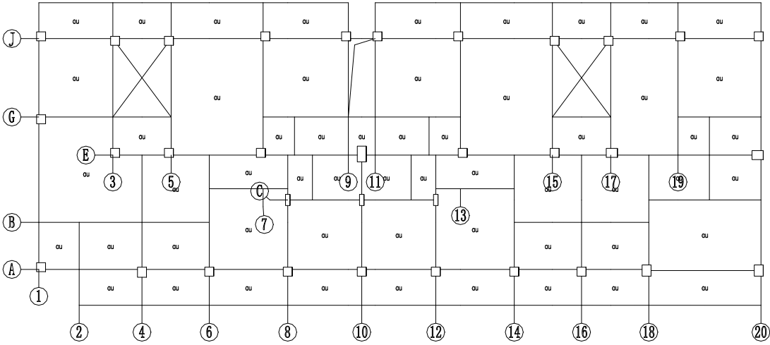
图 5.2.23 六层板安全评级结果简图(抗力与荷载效应之比)
