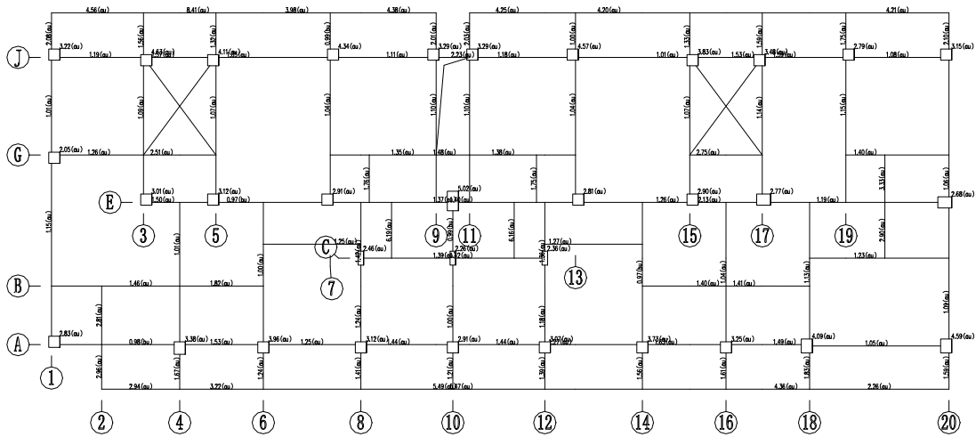
图 5.2.12 三层柱、四层梁安全评级结果简图 (抗力与荷载效应之比)
