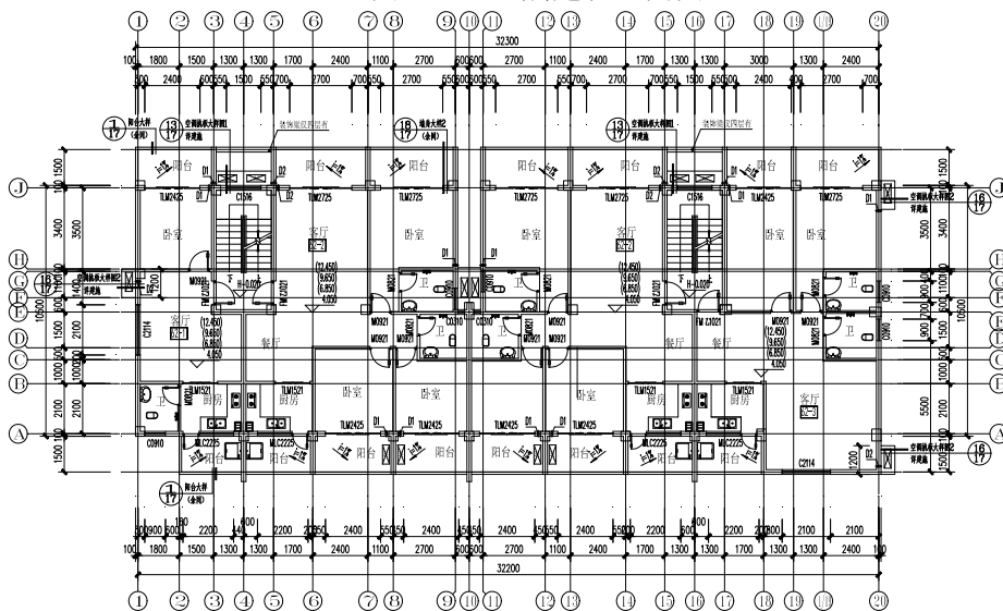
图 5.1.4 三层至六层建筑平面图
