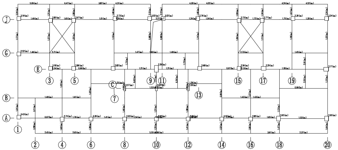
第 1 层 (标准层1) 构件评级结果简图 (承载力项)
