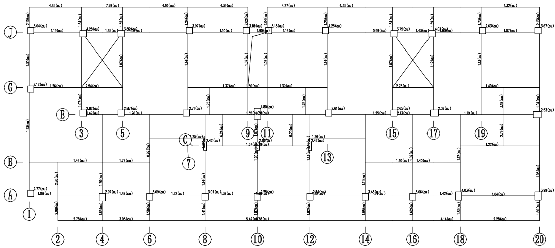
第 3 层 (标准层3) 构件评级结果简图 (承载力项)
