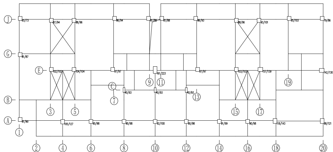
第 7 层 (标准层7) 抗震验算简图
