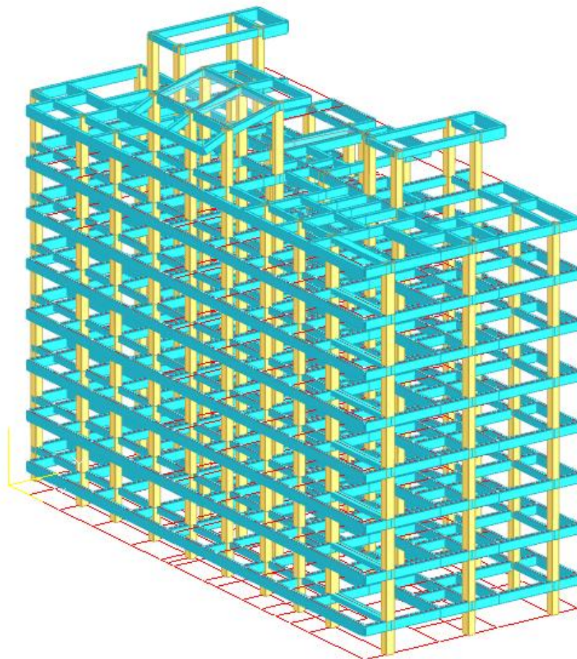
图 5.1.1 建模简图
