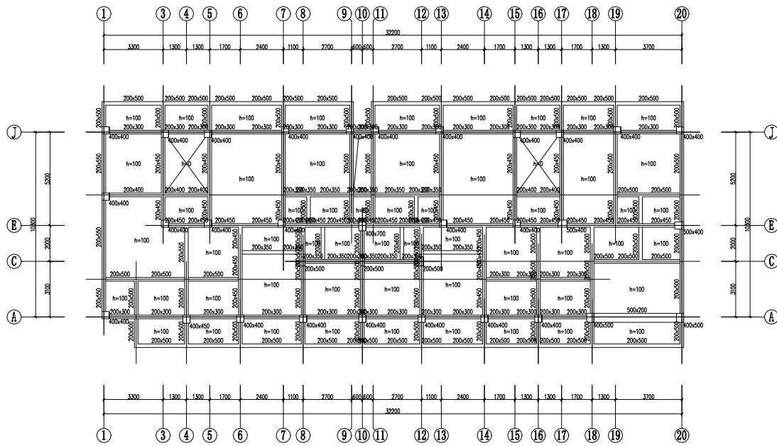
第5层 构件布置模版图(单位: mm)
