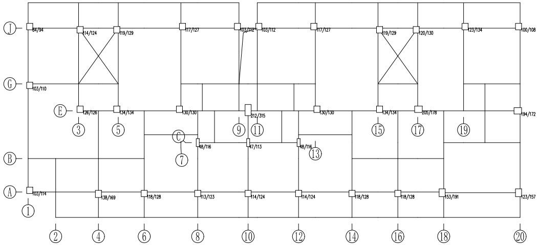
第 5 层 (标准层) 抗震承载力计算图 图号: 1 X 向 屈服强度系数=18.2 抗震能力指数=18.2 Y 向 屈服强度系数=22.8 抗震能力指数=22.8
