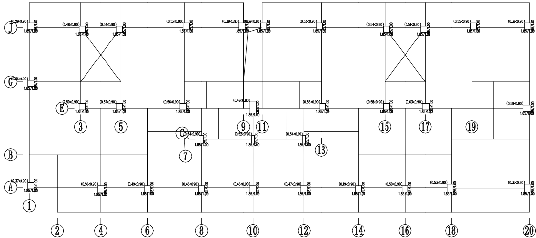
第1层(标准层1)柱、墙轴压比与长度系数简图
