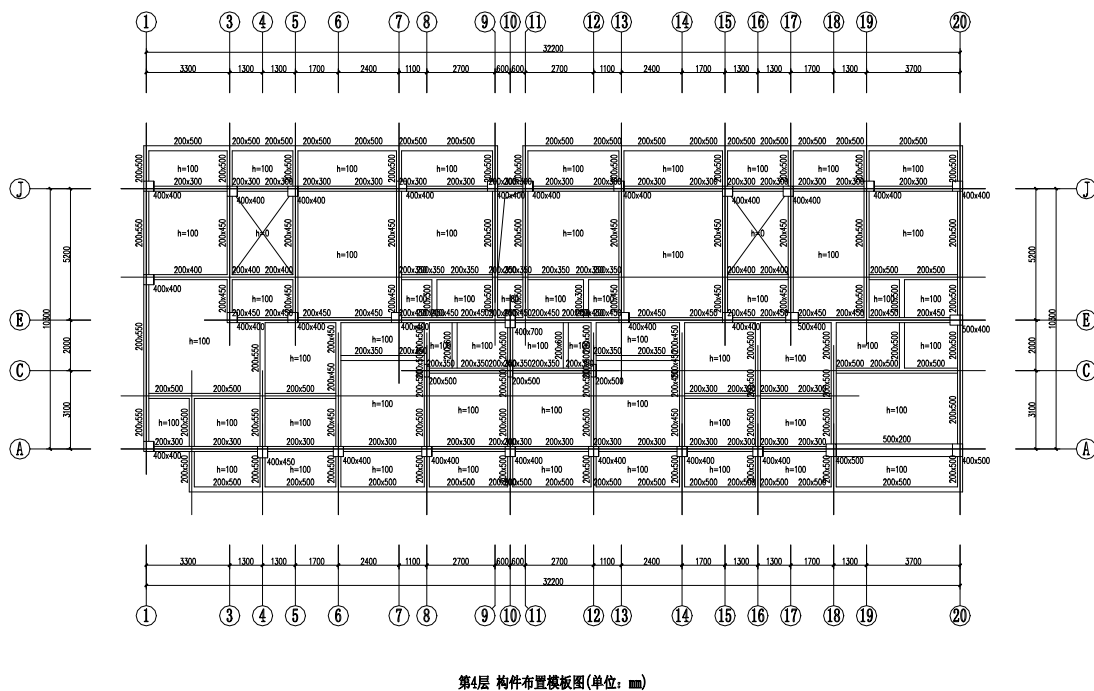
图 5.1.11 五层结构平面图
