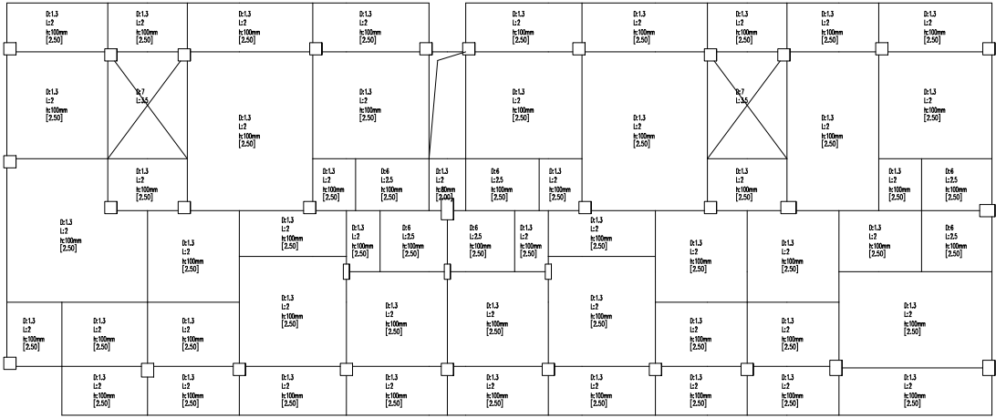
图 5.3.5 五层荷载平面简图
