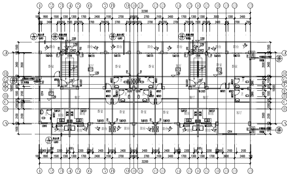
图 5.1.3 二层建筑平面图
