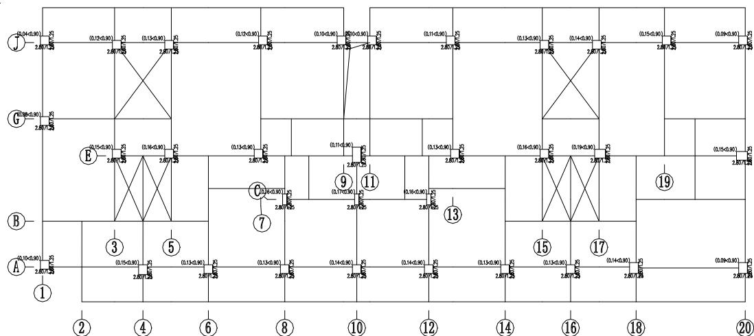
图 5.2.6 六层轴压比简图
