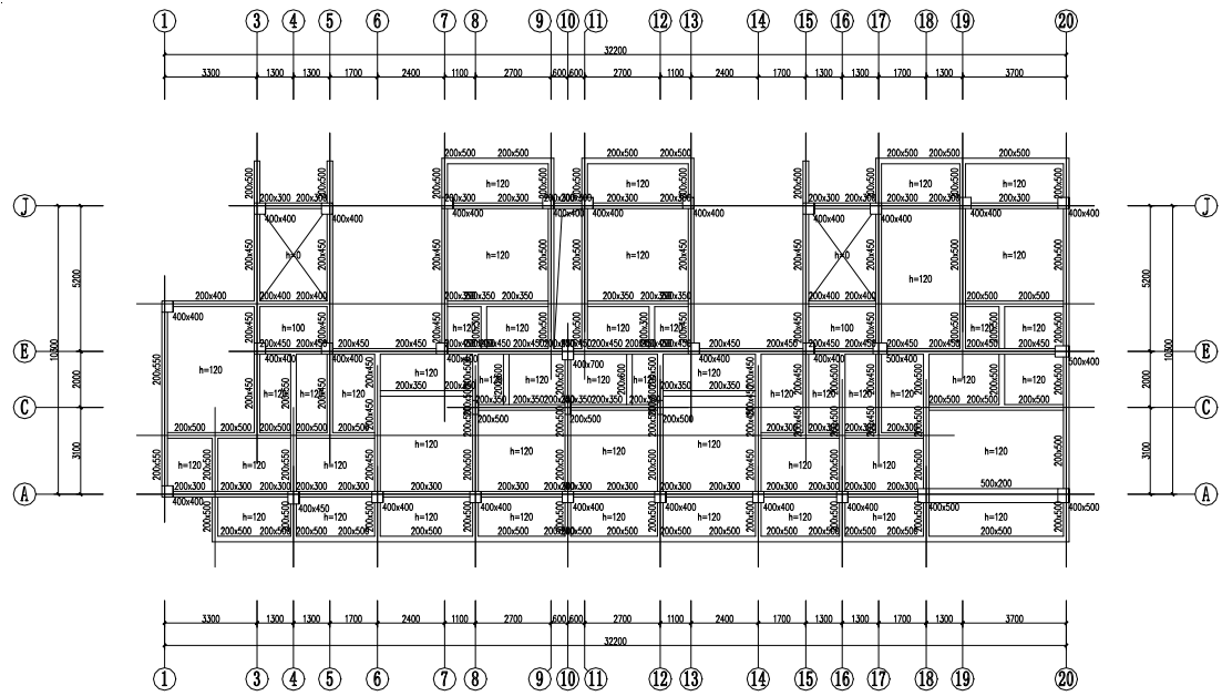
图 5.1.13 八层结构平面图
