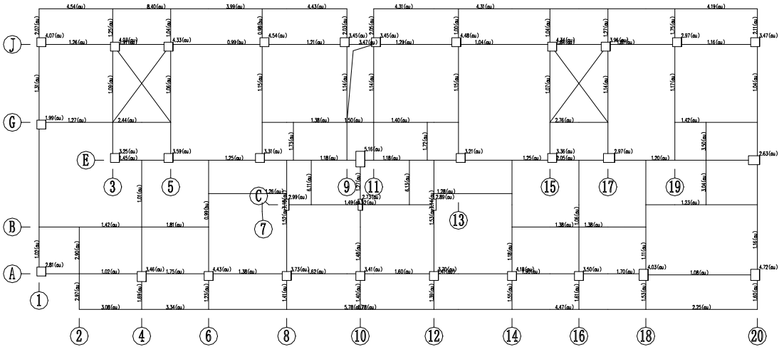
图 5.2.14 五层柱、六层梁安全评级结果简图 (抗力与荷载效应之比)
