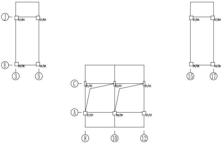
第 9 层 (标准层) 抗震承载力验算 层号: 1 X 向 层间刚度系数=33.4 抗震能力指数=33.4 Y 向 层间刚度系数=38.1 抗震能力指数=38.1
