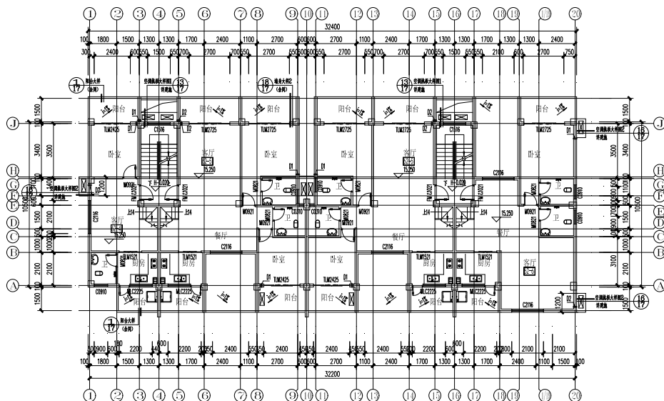
图 5.1.5 七层建筑平面图
