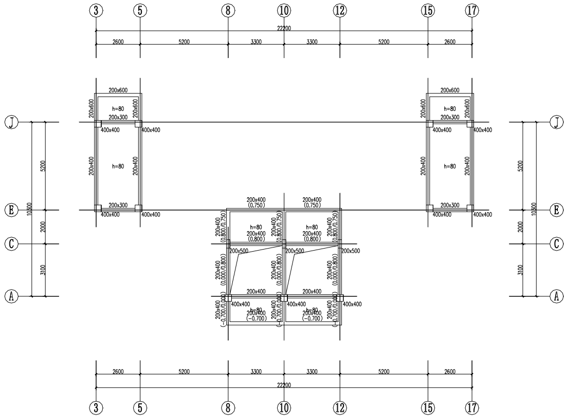
第9层 构件布置模板图(单位: mm)
