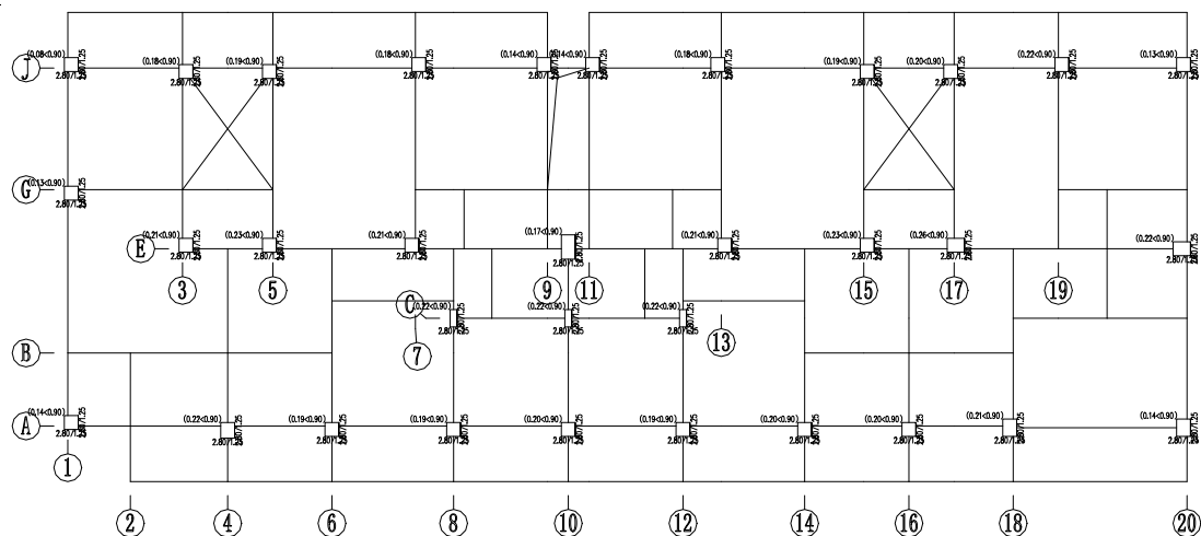
第6层(标准层6)柱、墙轴压比与长度系数简图
