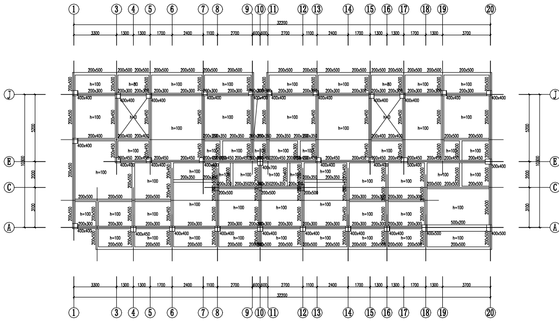
第1层 构件布置模板图(单位: mm)
