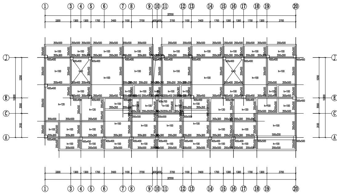
第6层 构件布置模版图(单位: mm)
