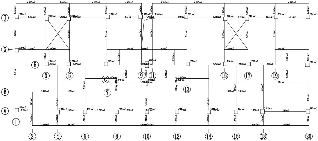
图 5.2.10 一层柱、二层梁安全评级结果简图 (抗力与荷载效应之比)
