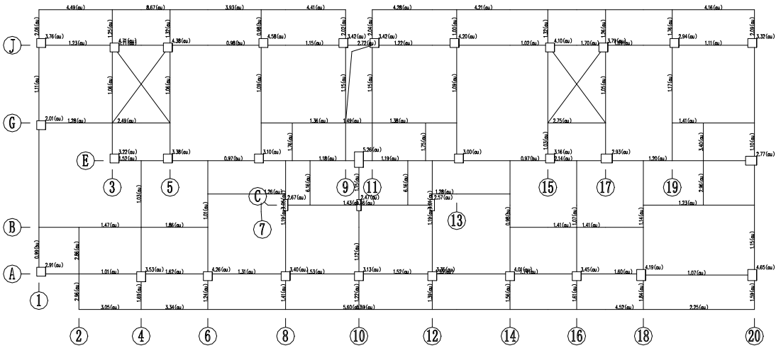
第 5 层 (标准层5) 构件评级结果简图 (承载力项)
