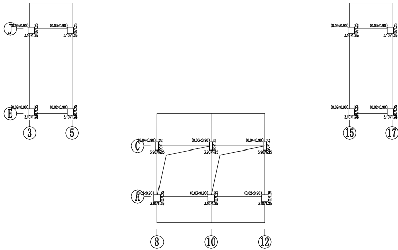
第 9 层 (标准层9) 柱、墙轴压比与长度系数简图
