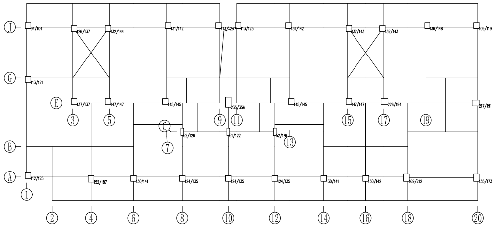
图 6.3.3 三层抗震验算结果
