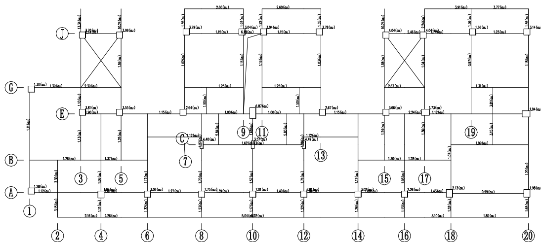
图 5.2.16 七层柱、屋顶构架层梁安全评级结果简图 (抗力与荷载效应之比)
