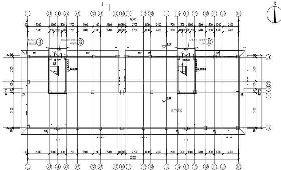
图 5.1.2 一层建筑平面图
