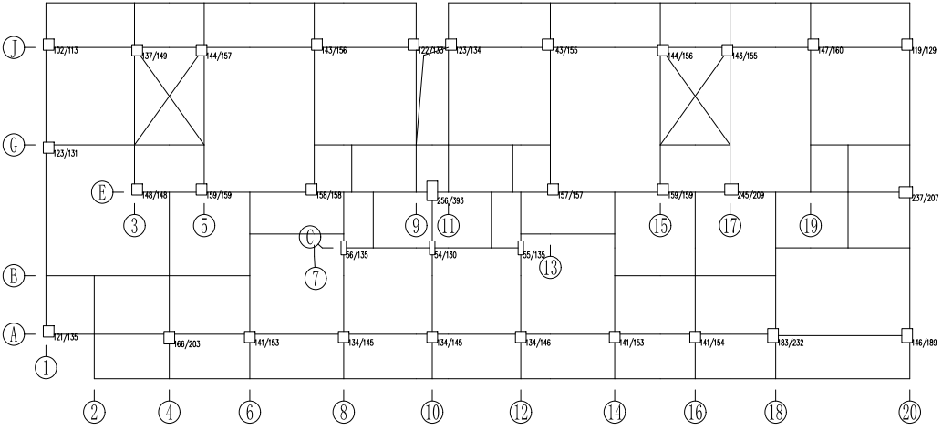
第 3 层 (标准层3) 抗震承载力验算 层数: 1 X向 屈服强度系数=17.4 抗震能力指数=17.4 Y向 屈服强度系数=22.0 抗震能力指数=22.0
