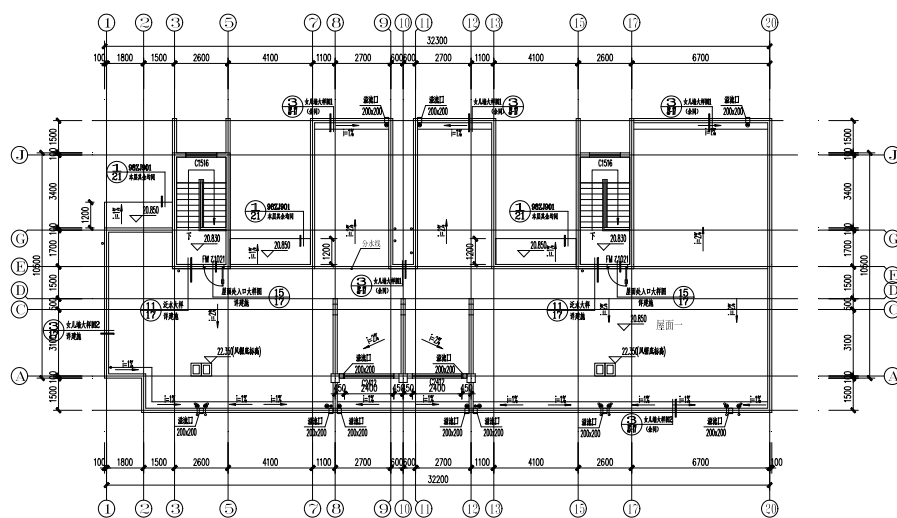
图 5.1.7 屋面层建筑平面图
